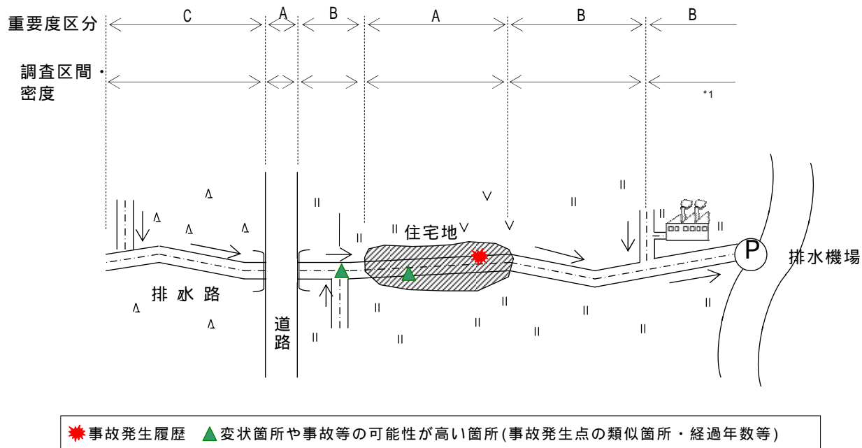
図 2-5 調査地点・調査密度の設定の例（排水系）
