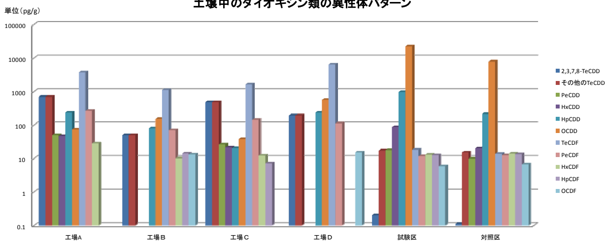
図3 パルプ工場排水から遠心分離された浮遊物中及び電解次亜塩素酸水を長期散布した土壌中のダイオキシン類の異性体パターン
