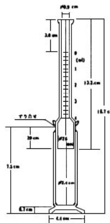
第2図 ガス定量器
