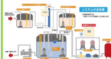
排液リサイクルシステム
