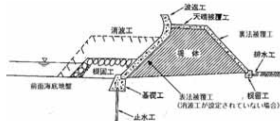
堤 防
