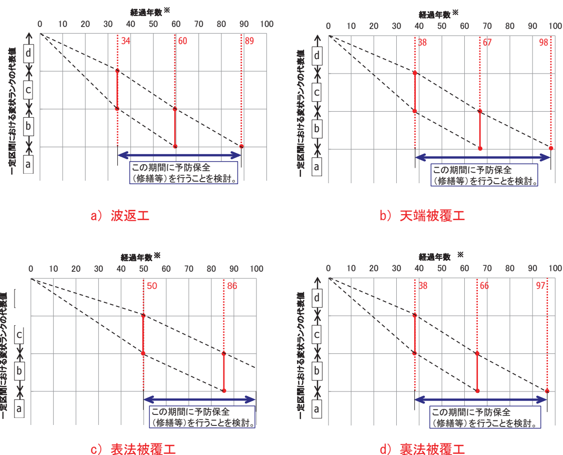
図-6.7 護岸の場合の部材ごとの劣化予測と修繕等の時期
