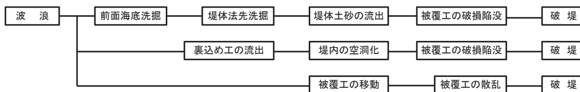
図-5.6 護岸・堤防の進行型変状連鎖
