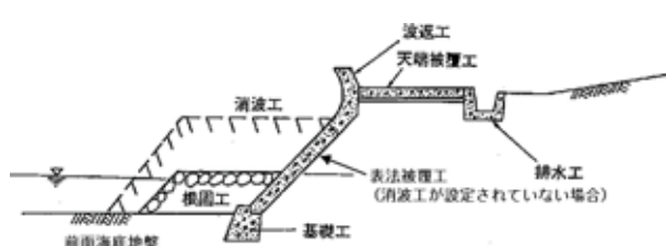
護 岸
