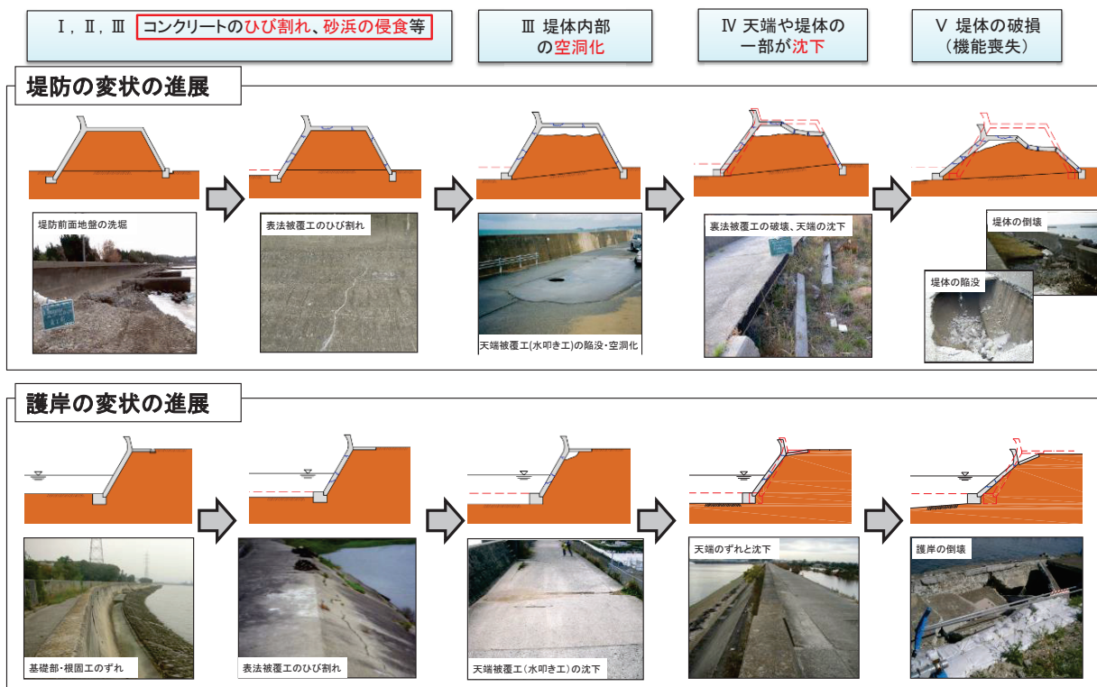
図-2.5 変状の進展の具体例
