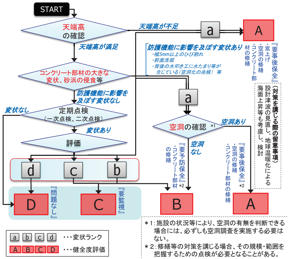
図-5.3 健全度評価のフロー
