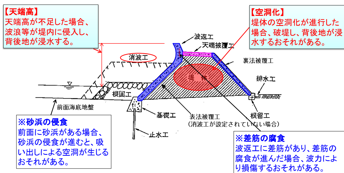
図-2.3 断面における点検の重要な視点のイメージ
