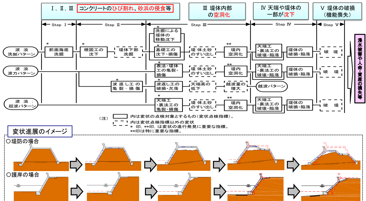
図-2.4 変状連鎖における点検の重要な視点のイメージ
