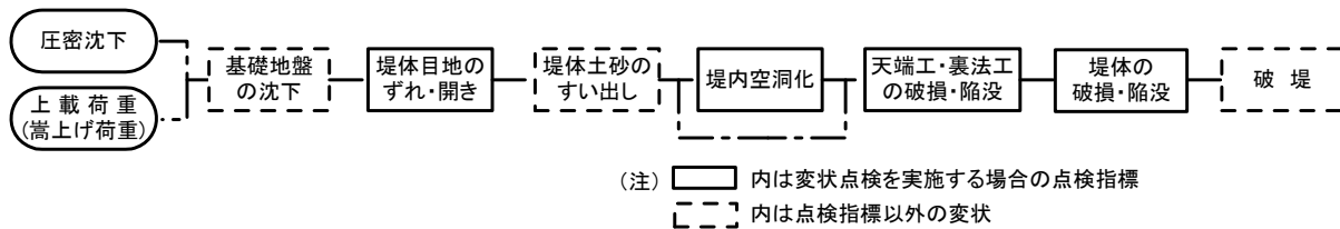
図-5.6 護岸・堤防の進行型変状連鎖
