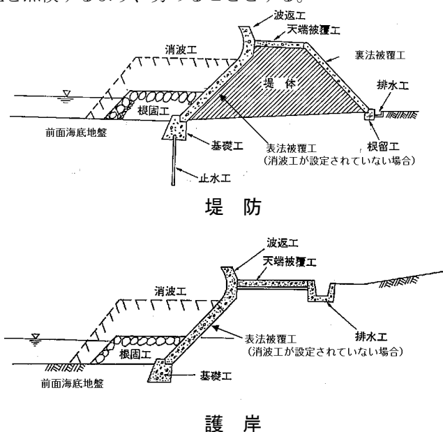
図-2.6 海岸保全施設の点検位置
