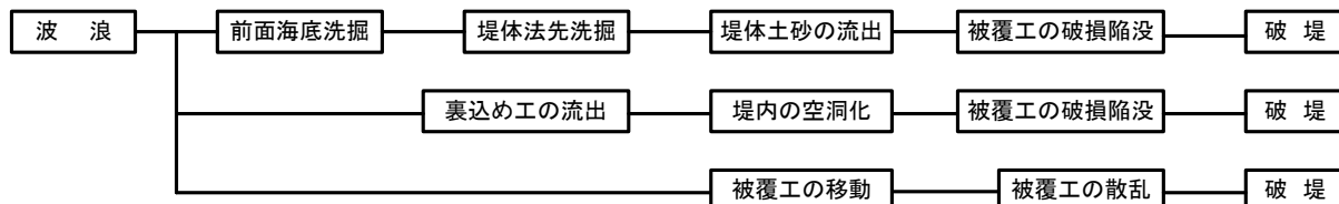
図-5.6 護岸・堤防の進行型変状連鎖
