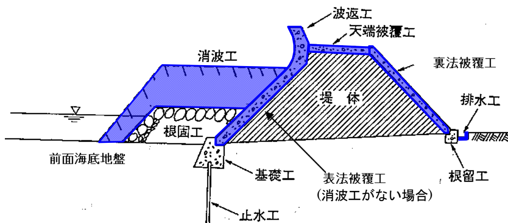
図-5.2 堤防等の健全度評価を行う主な箇所
