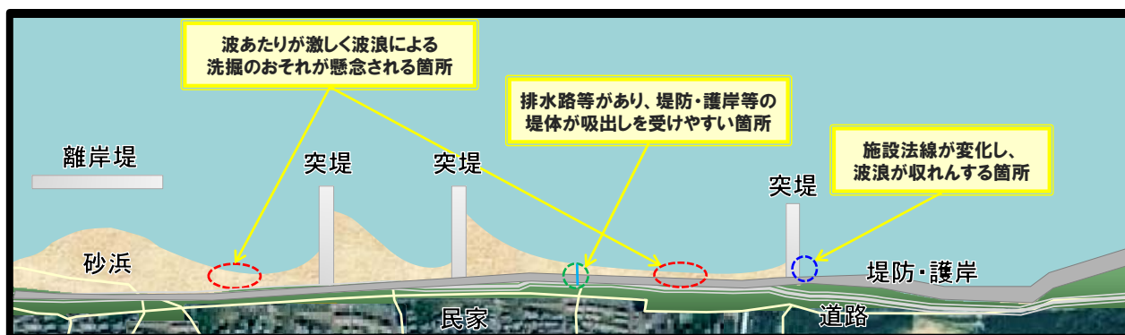
図-2.2 地形等により劣化や被災による変状が起こりやすい箇所のイメージ
