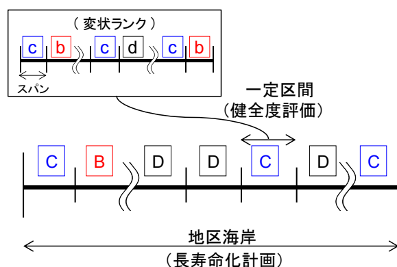
図-5.1 一定区間とスパン(イメージ)
