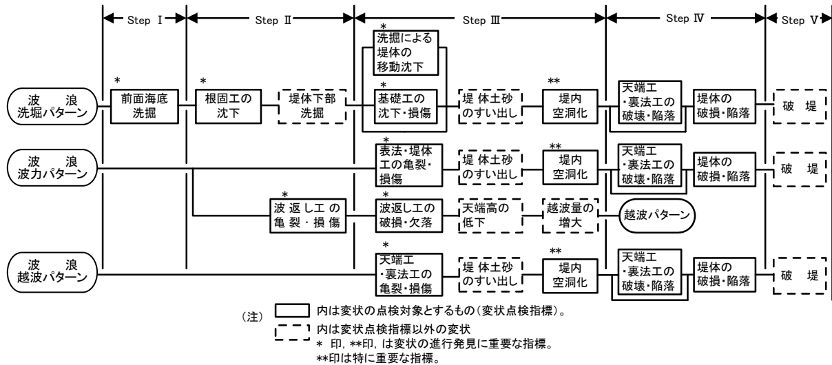
図-5.4 堤防(消波工なし)の主要変状連鎖
