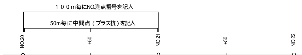
図 2-1 平面線形の表現方法
