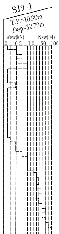
図 3-11 スウェーデン式サウンディング結果の記載例
