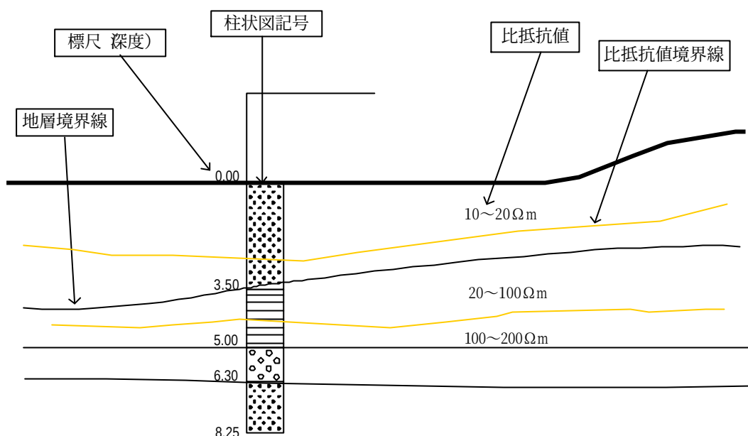
図 3-14 比抵抗断面図の記載例
