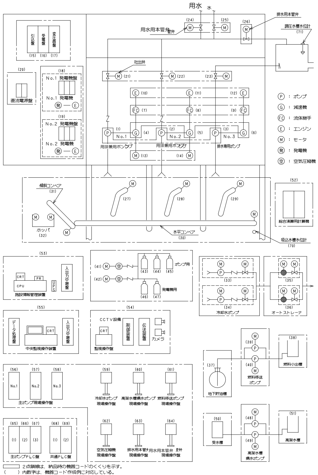
図 10-7 用排水ポンプ設備の構成図
