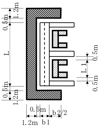
② 平面図
