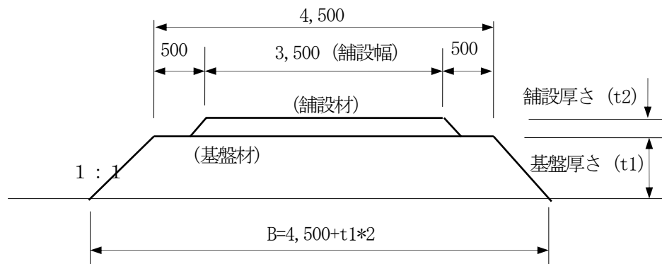
図15-17 標準断面図
