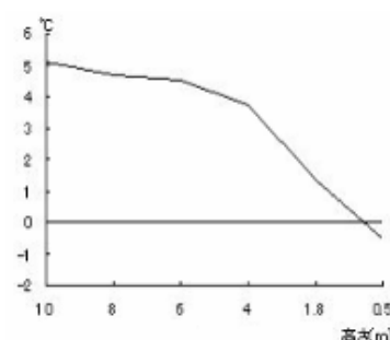
(図1) 逆転層の出現状況(小松1994)
