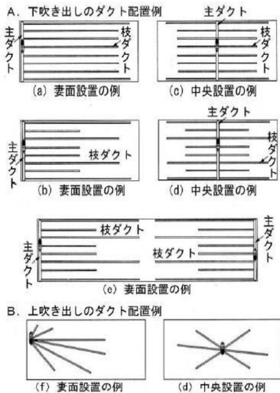
図－10 温風ダクトの設置方法
