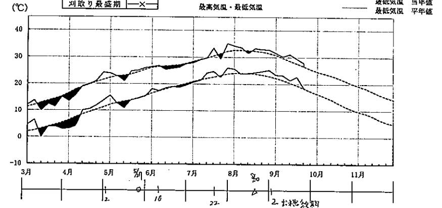
気温日較差
