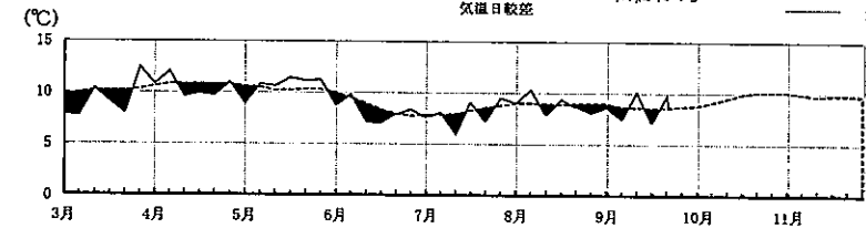
気温日較差
