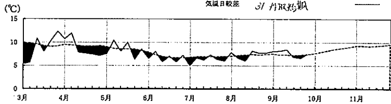
気温日較差
