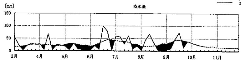
降水量
