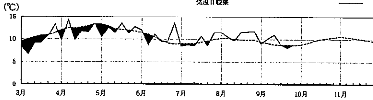
気温日較差
