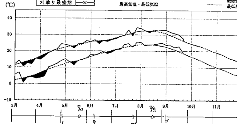
気温日較差
