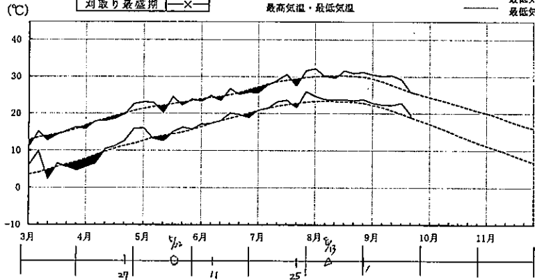
気温日較差
