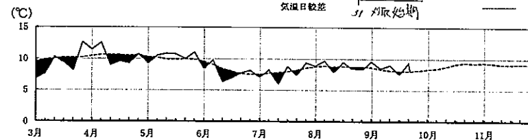
気温日較差
