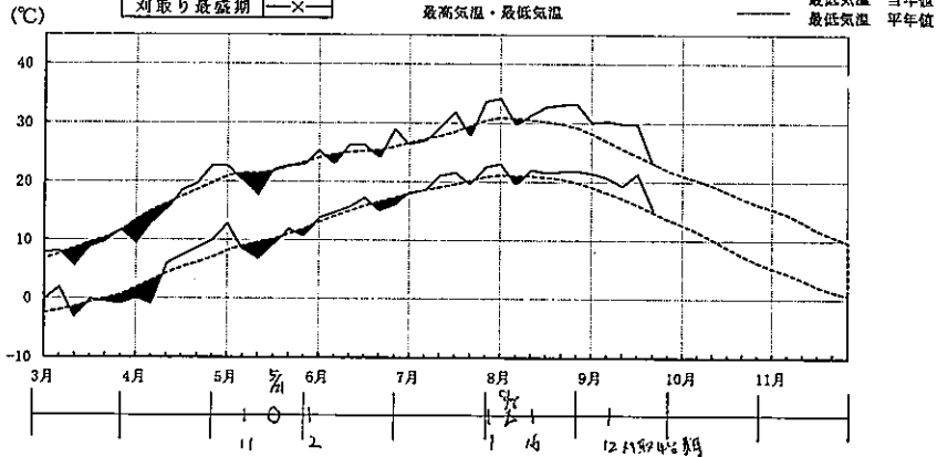
気温日較差
