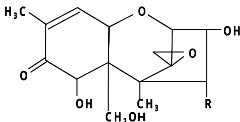
DON (R=H) 及びNIIV (R=OH) の化学式
