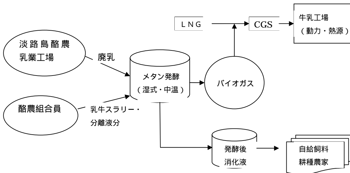
バイオメタンガスコジェネシステム
