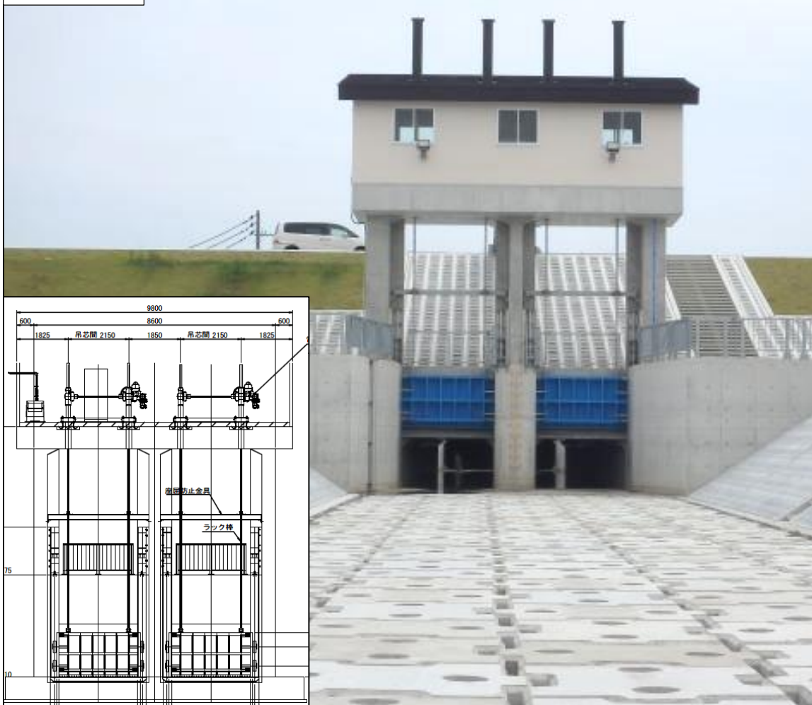
新排水樋門
