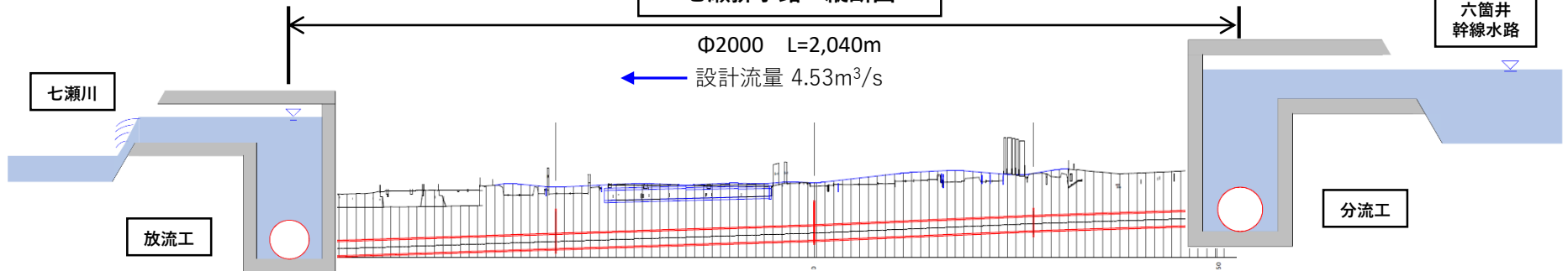
七瀬排水路 縦断図
