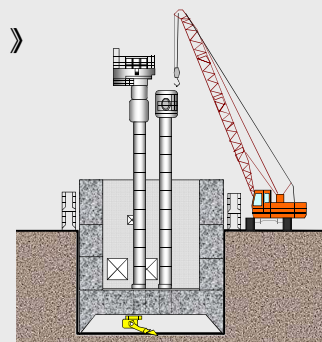
ニューマチックケーソン工法施工断面図
