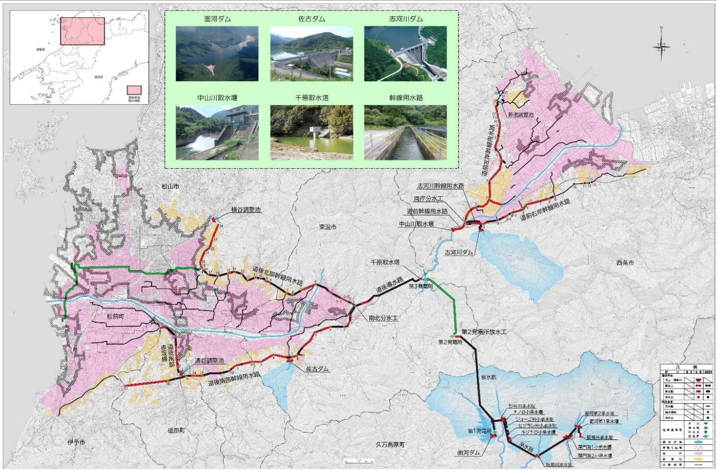
道前道後用水農業水利事業 計画一般平面図
