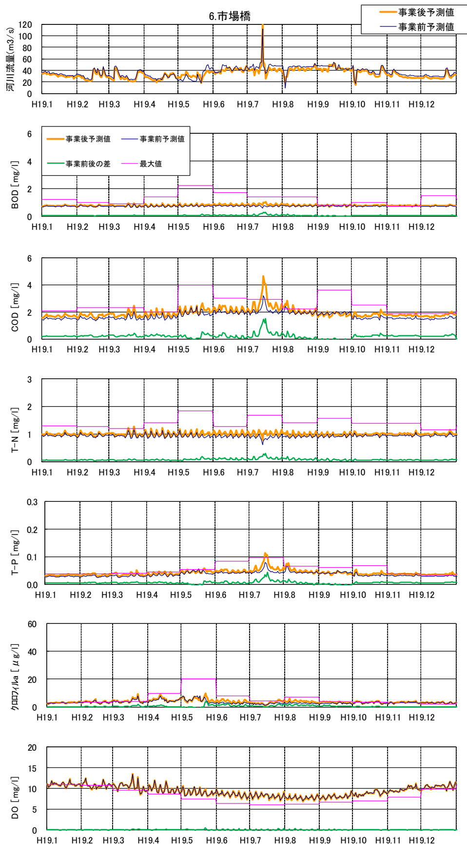
図 1-2 (6) 事業前後の水質予測結果 (H19 渇水年)
