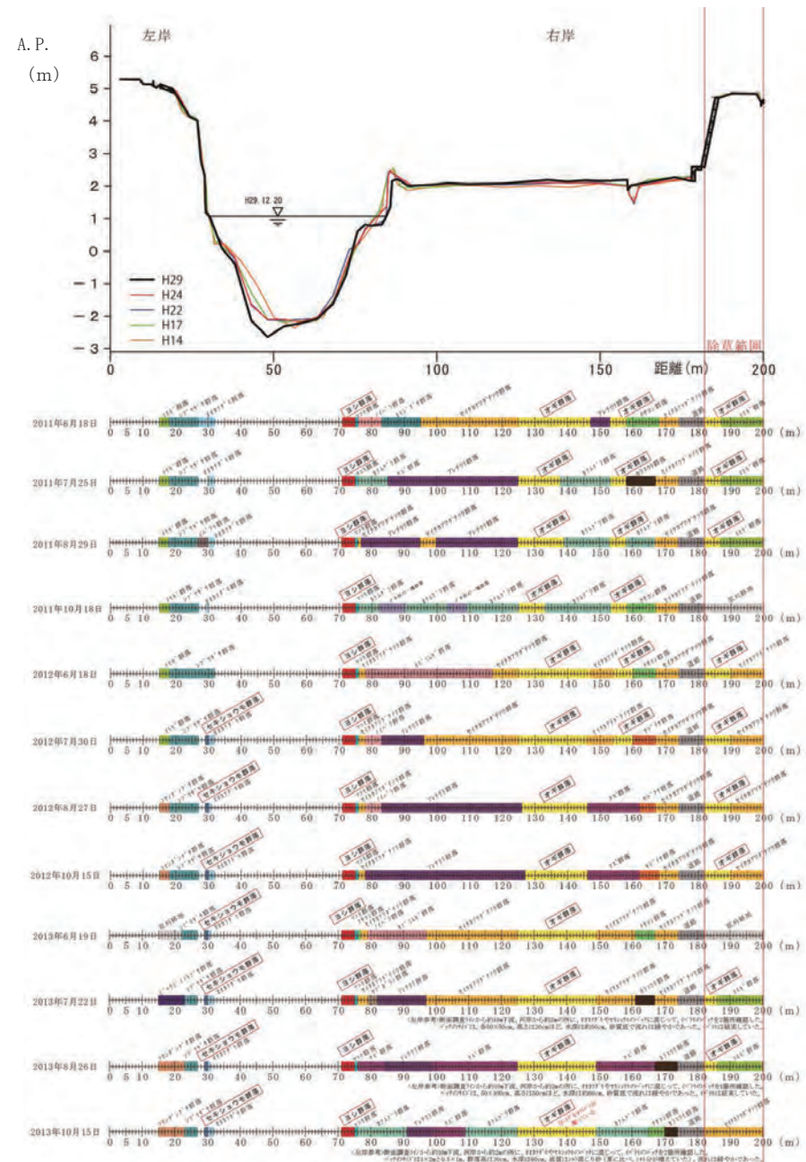
図 2. 6. 7. 2 (4) 植生断面図の変化 (旧吉野川 18.6 km地点)
