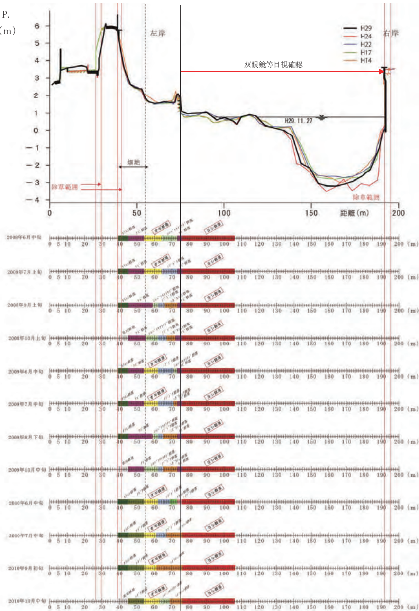
図 2.6.7.4(3) 植生断面図の変化（今切川 11.4 km地点）
