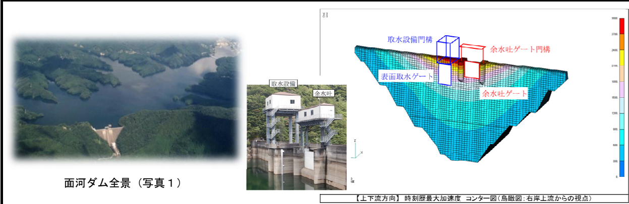
堤体の全体3次元モデルによる動的解析（図1）
