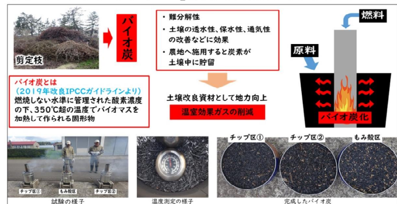
図1 バイオ炭製造試験の様子
