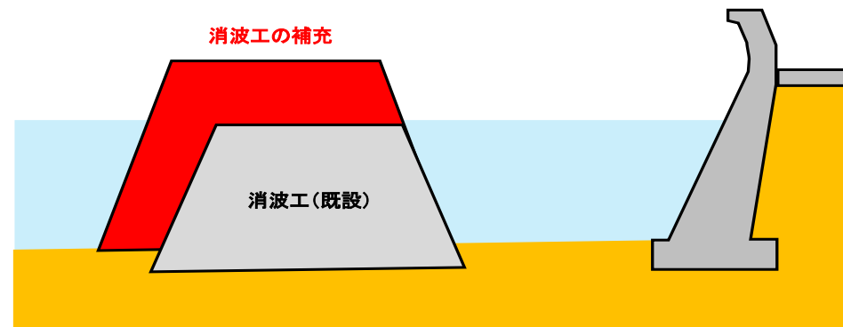
消波工の補充(消波断面の回復)
