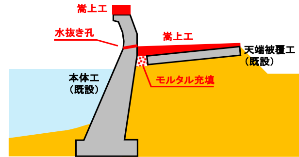
嵩上げ工法(既設構造物を使用) 水抜き孔の削孔 モルタル充填(機能回復)
