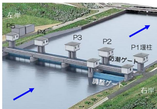
河北潟防潮水門完成イメージ図
