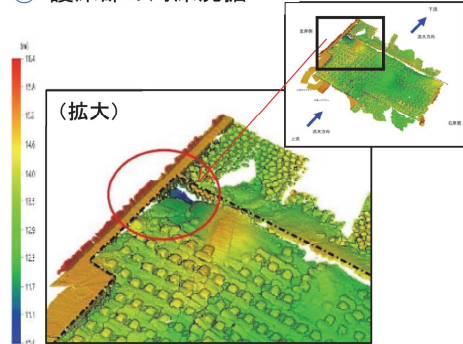
② 護床部の河床洗掘
