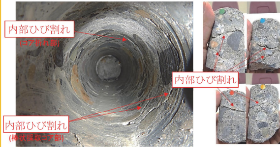
③ 堰柱コンクリートの内部ひび割れ
