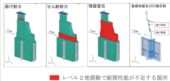
④ 頭首工の耐震性能不足
