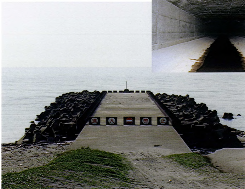
国上隧道河海工完成 (平成15年4月撮影)
