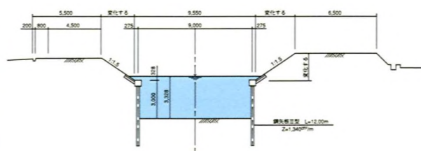
標準断面図(1号)
