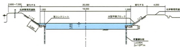
標準断面図(第1号)
