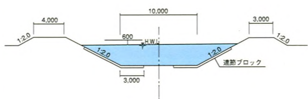
上流部標準断面図(2号)
