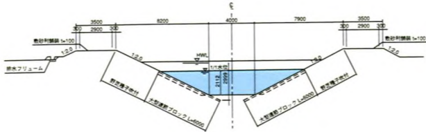
ブロック護岸標準断面図(4号単断面)
