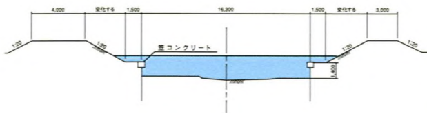
標準断面図(第1-1号)
