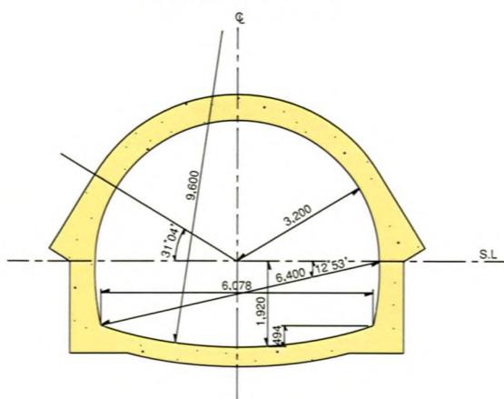
国上隧道標準断面図
