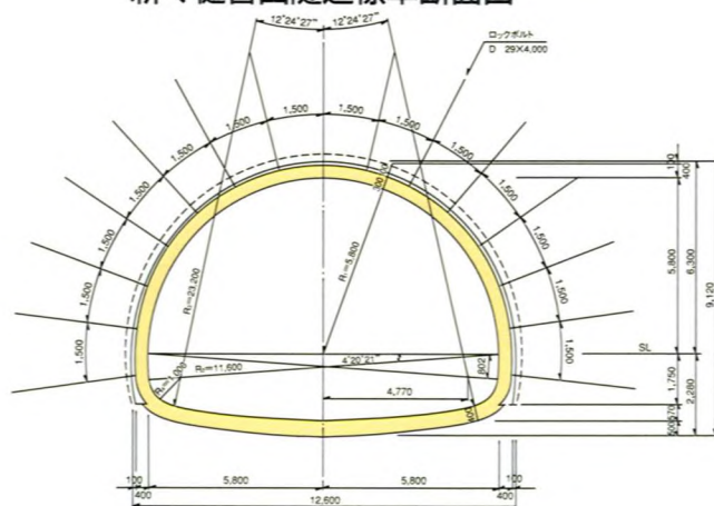
新々樋曾山隧道標準断面図
