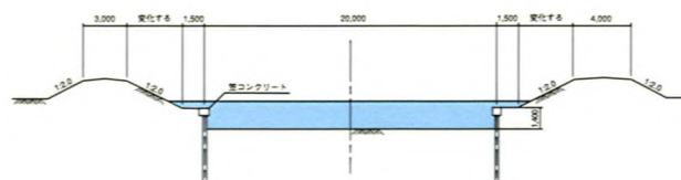
標準断面図 (第1号)
