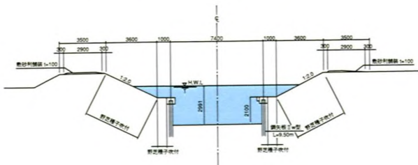
鋼矢板護岸標準断面図(4号複断面)
