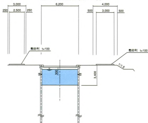
標準断面図(第4号)
