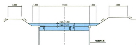
標準断面図
