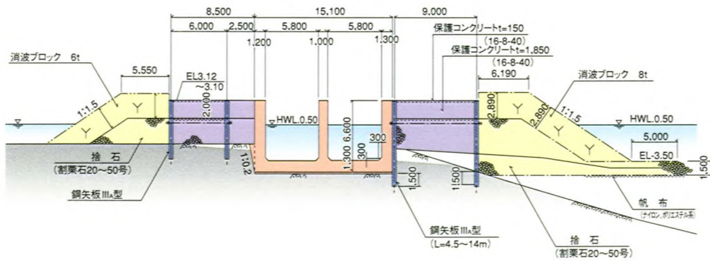
新々樋曾山隧道 河海工標準断面図
