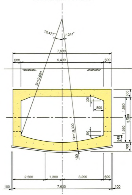
野積暗渠標準断面図
