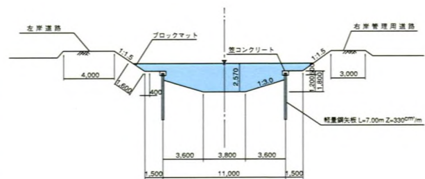
支線標準断面図
