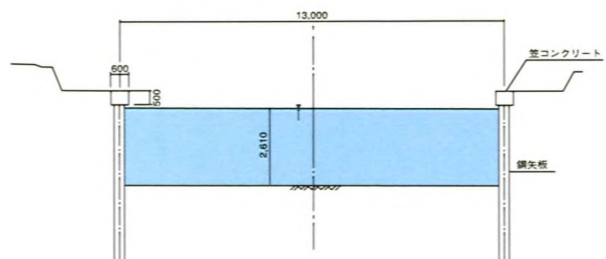
下流部標準断面図
