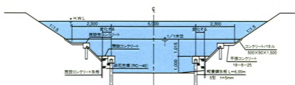
標準断面図
