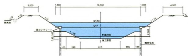
標準断面図 (2号)
