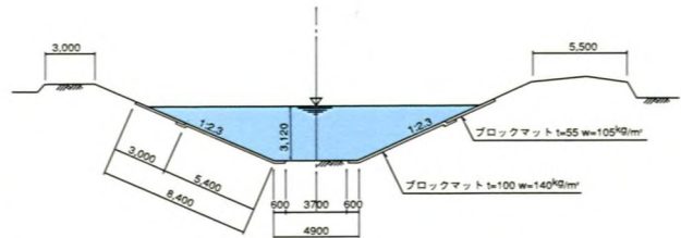
幹線標準断面図(第2-1号)
