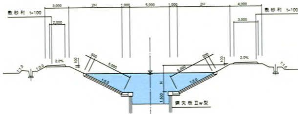
標準断面図(第1-1号)
