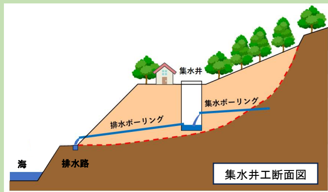
【本復旧（集水井イメージ図・写真）】
