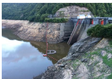
内の倉ダムの渇水状況 （平成30年）
