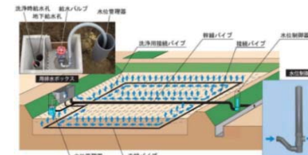
地下かんがい
