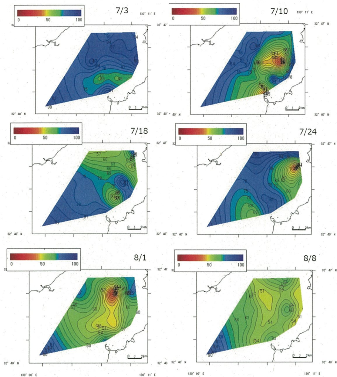
図 2-1-6. 底層(B-1)DO(%)7/3-8/8 の推移
