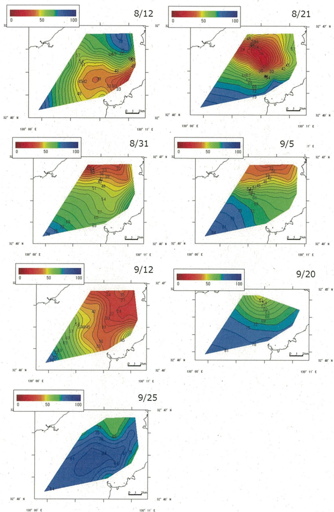
図 2-1-6. 底層(B-1)DO(%)8/12-9/25 の推移
