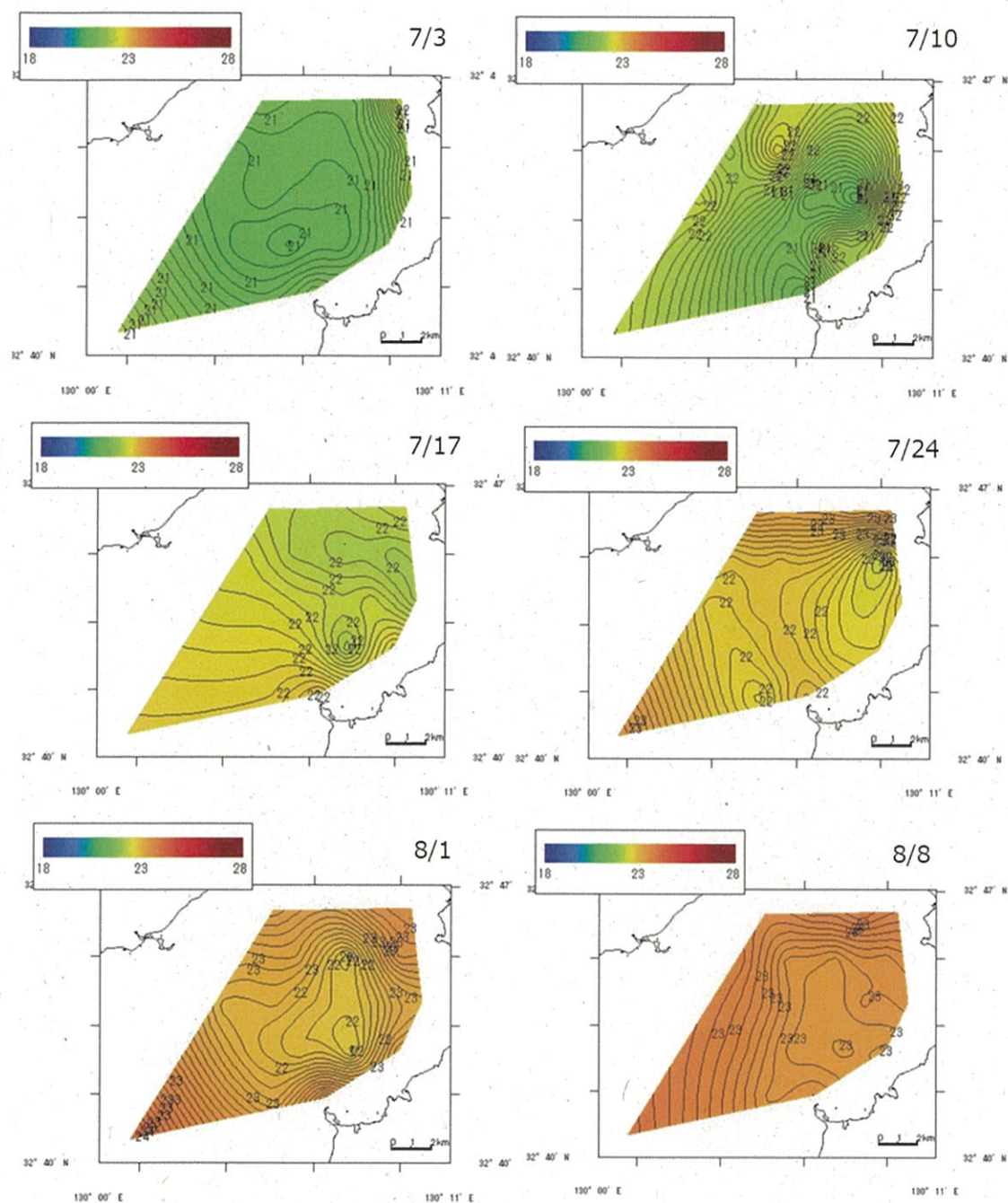
図 2-1-7. 底層(B-1)水温(°C) 7/3-8/8 の推移
