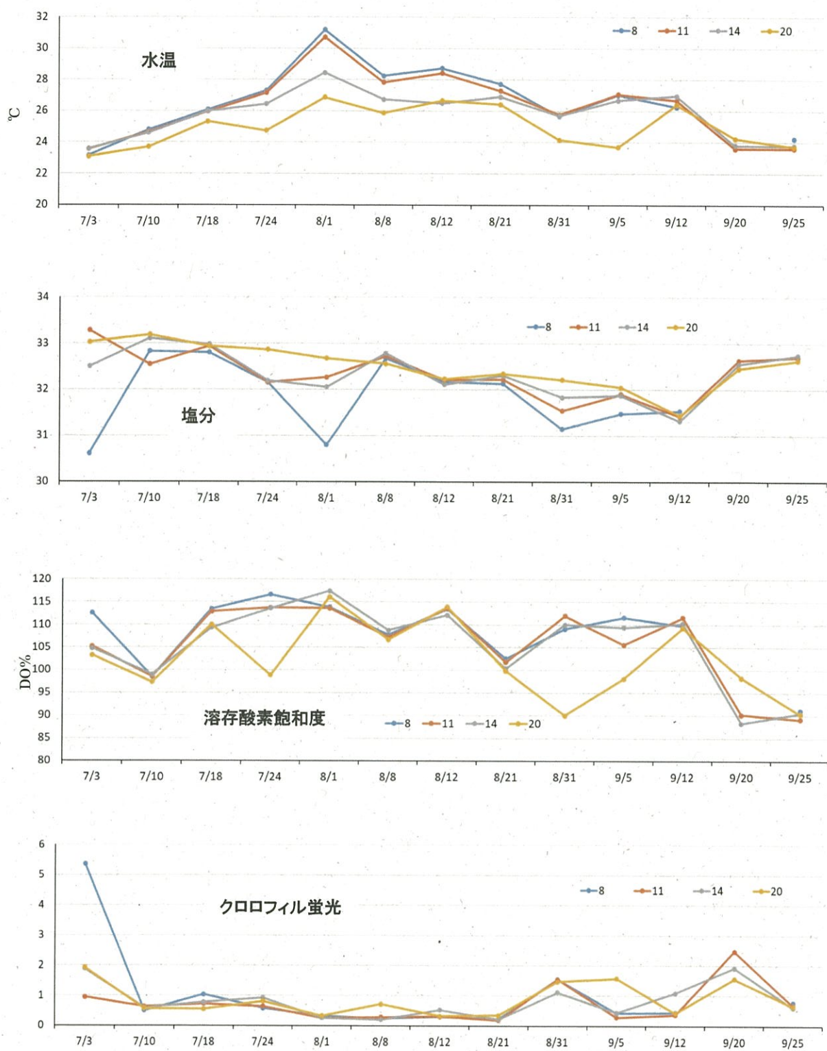
図 2-1-3. St.8、11、14、20 の表層水温、塩分、溶存酸素飽和度、クロロフィル蛍光の推移
