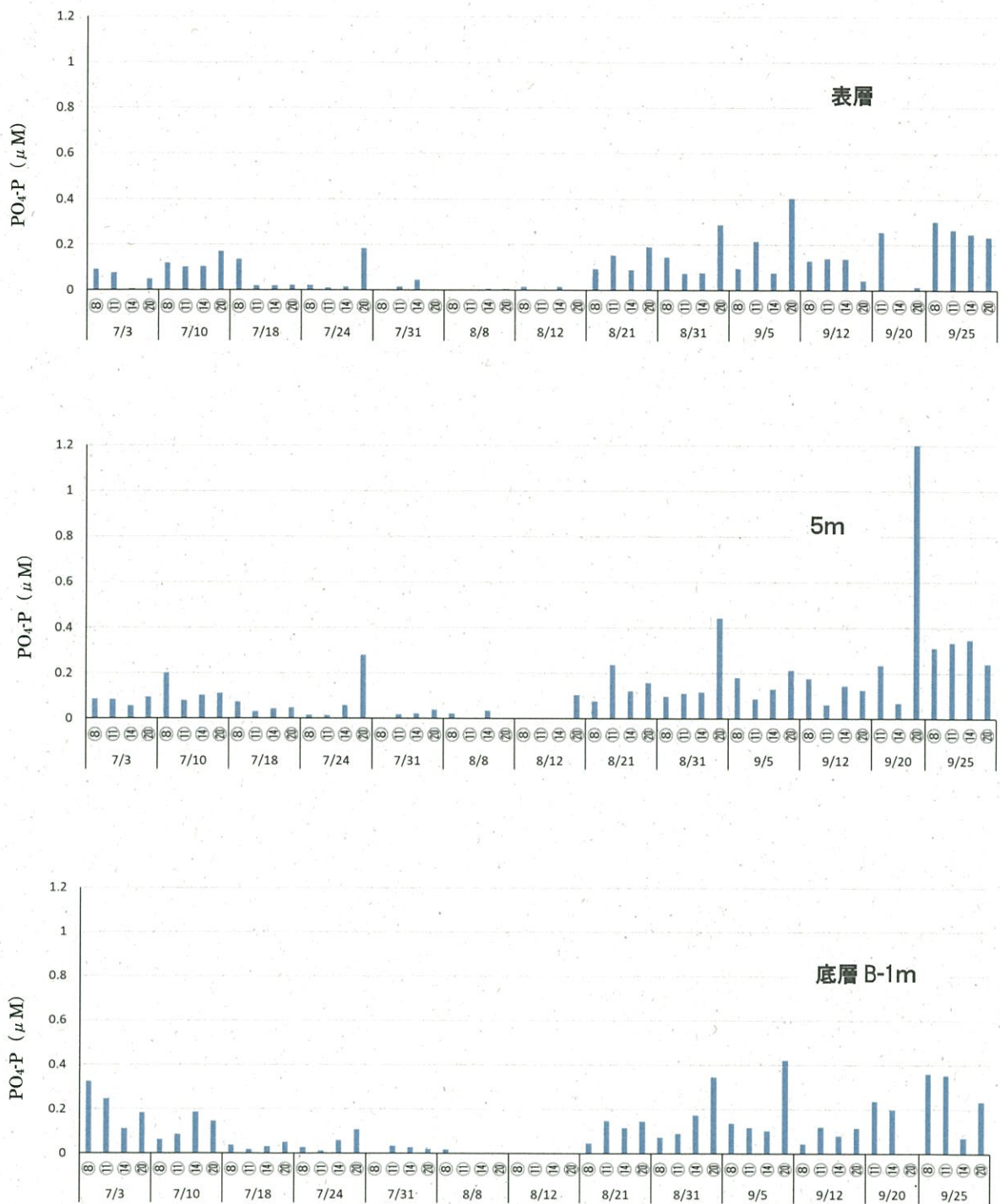
図 2-1-4. 調査点ごとの栄養塩濃度( PO_4-P )
