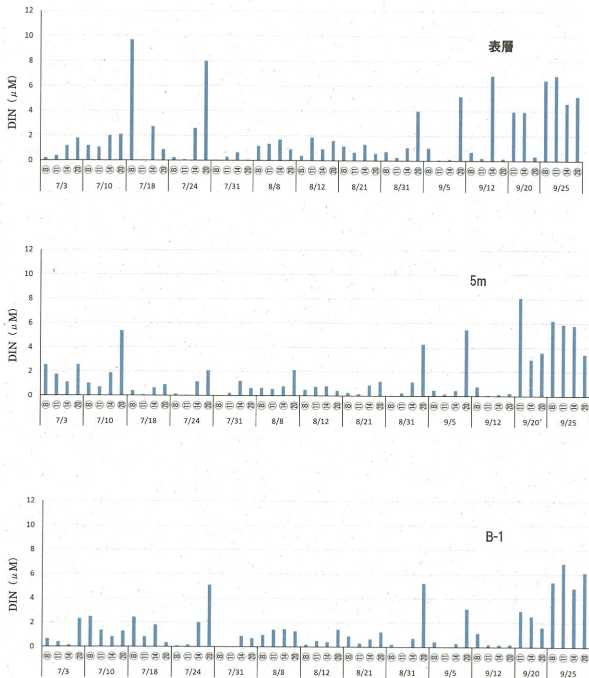
図 2-1-4. 調査点ごとの栄養塩濃度(DIN)
