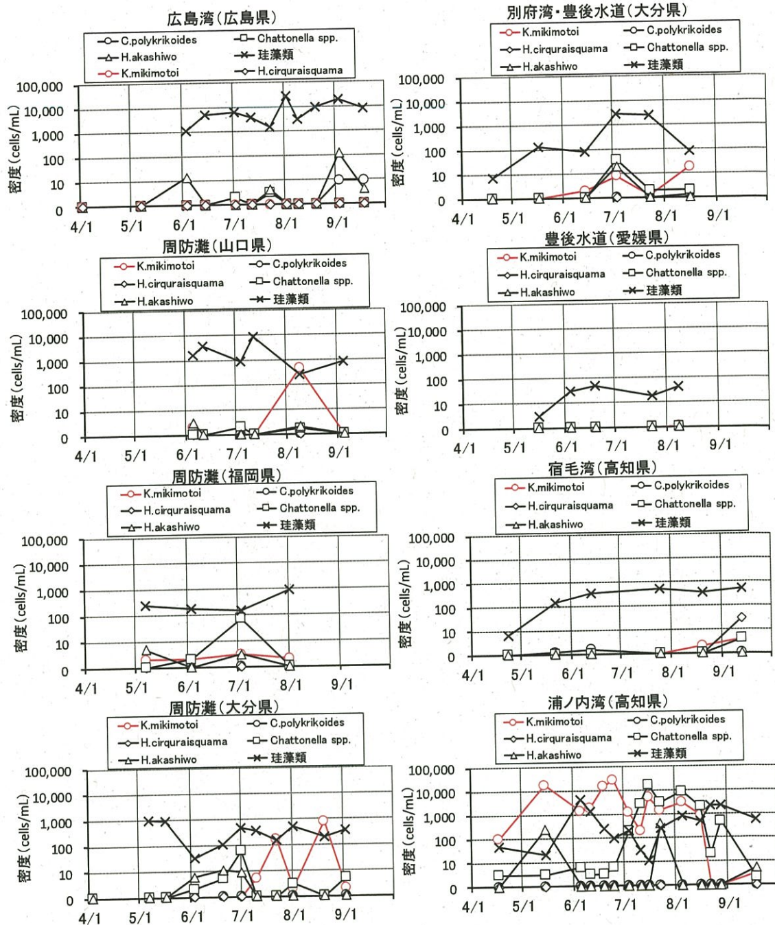
図 12 各県海域におけるプランクトン密度の推移 (有害種は最高密度, 珧藻類は表層平均密度)
