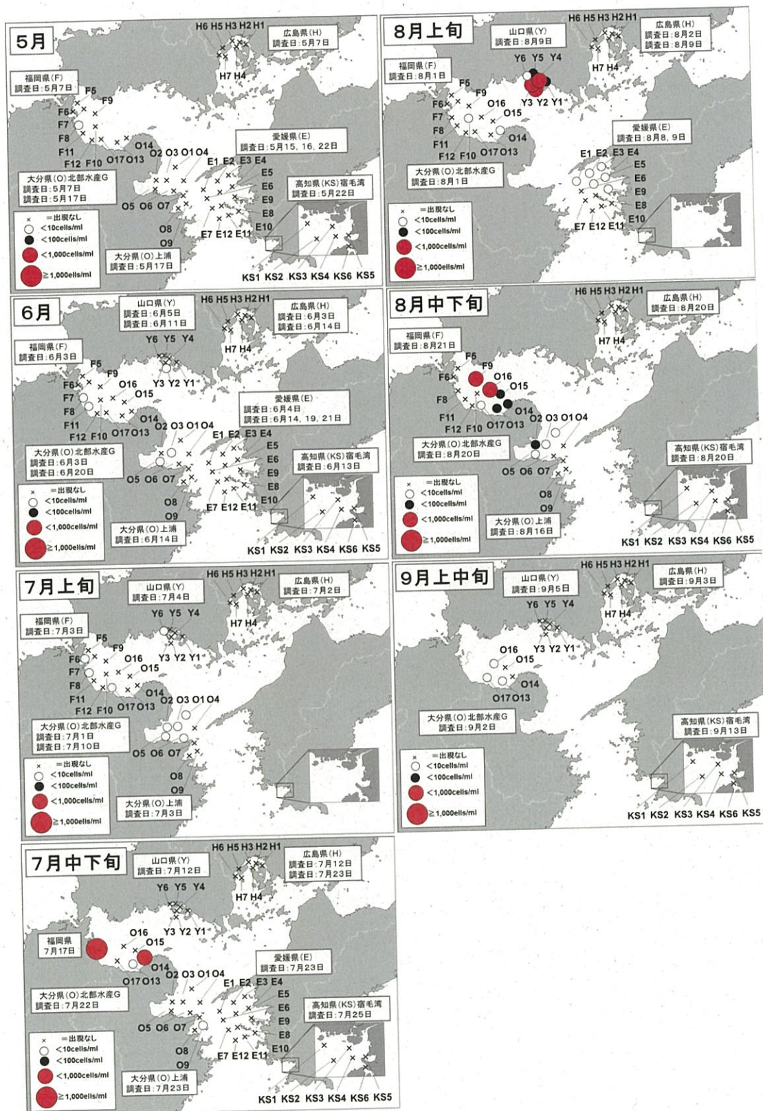
図 13 Karenia mikimotoi 細胞密度の水平分布 (広島湾, 周防灘, 別府湾, 豊後水道, 宿毛湾)
