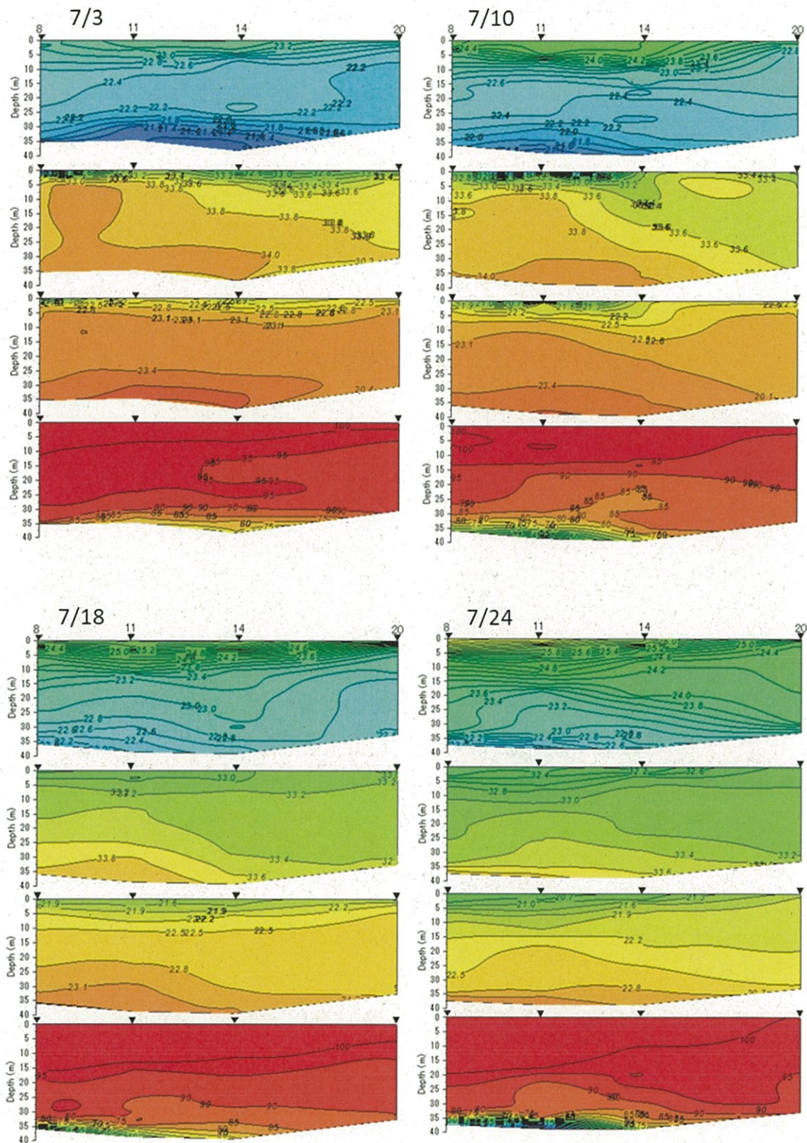
図 2-1-8. St.8, 11, 14, 20 における水温(°C)、塩分、 \sigma_t 、DO(%)の鉛直コンタ図(7/3-7/24)
