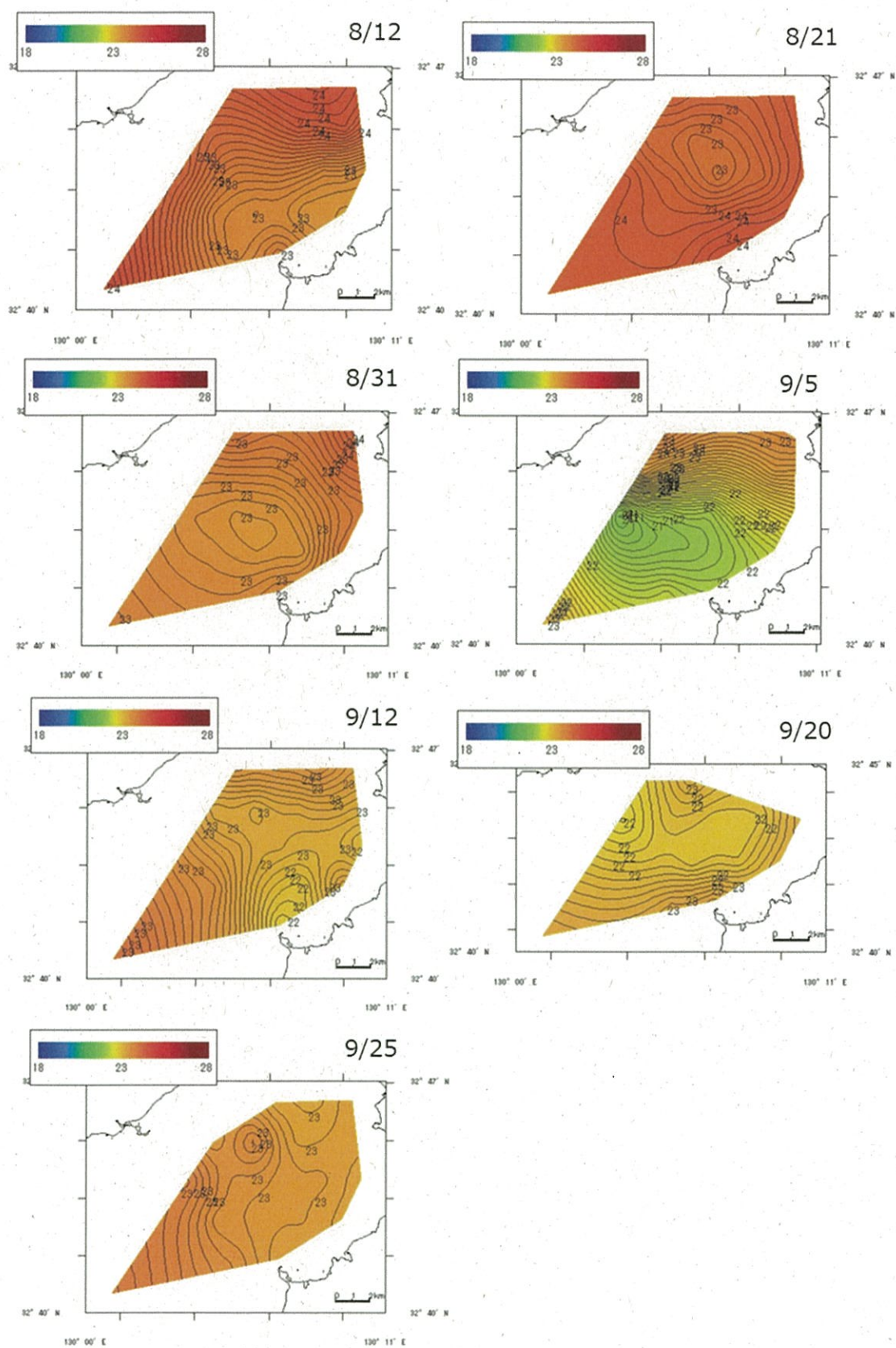
図 2-1-7. 底層(B-1)水温(°C) 8/12-9/25 の推移
