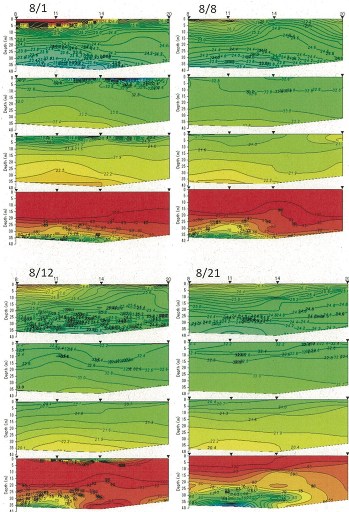
図 2-1-8. St.8、11、14、20 における水温(°C)、塩分、 \sigma_t 、DO(%)の鉛直コンタ図(8/1-8/21)
