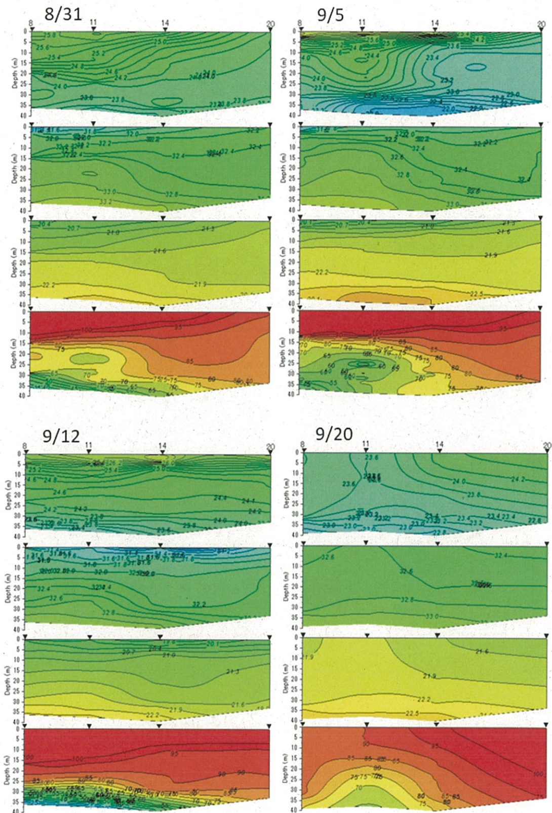
図 2-1-8. St.8、11、14、20 における水温(°C)、塩分、 \sigma_t 、DO(%)の鉛直コンタ図(8/31-9/20)
