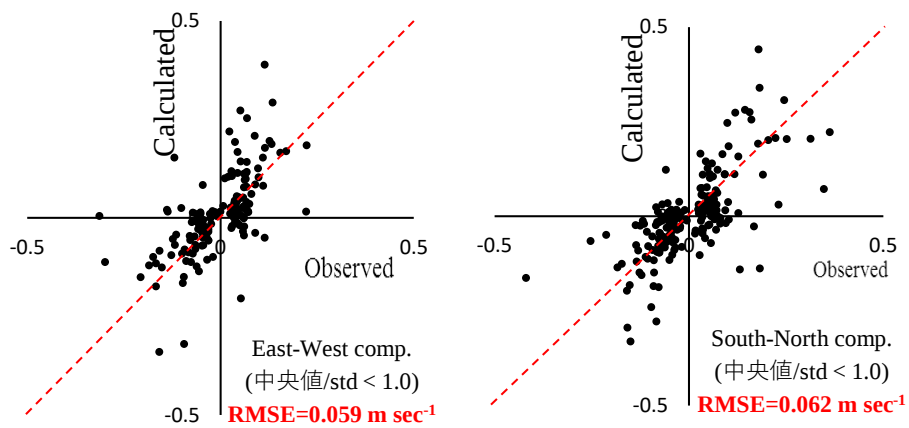
図 42-4 漁船搭載の ADCP による測流データと UCHI の比較 (左図:東西成分 右図:南北成分)
