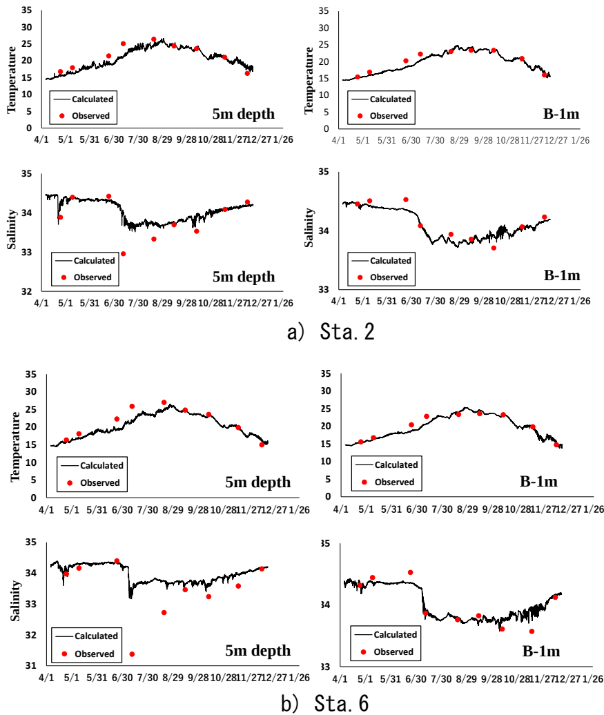
図 42-5 伊万里湾における水温・塩分の比較結果 (a:Sta.2 b:Sta.6)
