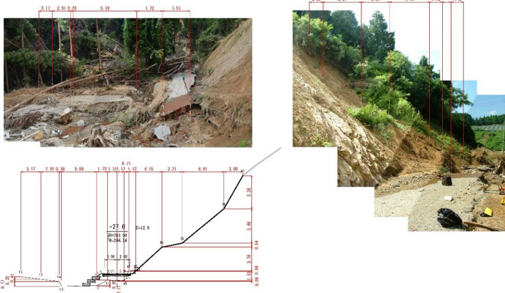
写真 2-17 平成 29 年災害 福岡県 同一路線において発生した複数の被災地
