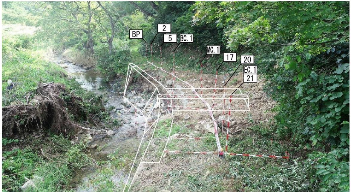
写真 2-13 平成 30 年災害 山形県 路体侵食
