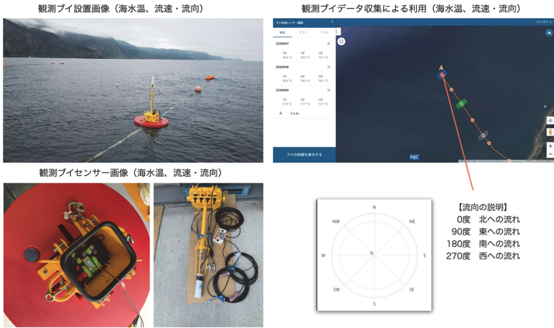
図 3 - 3 - 2 観測ブイ画像 (海水温 3 層・流向・流速)
