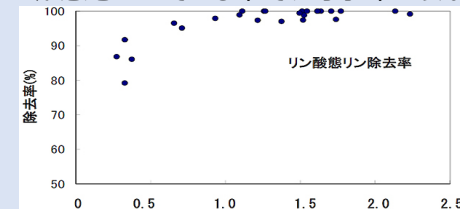
非晶質珪酸カルシウム水和物の添加率(kg/t)とりん除去率の関係
