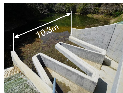
豪雨対策（洪水吐きの改修）の先行整備（例） ※地震対策は豪雨対策完了後に実施
