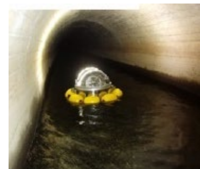
点検ロボットによる 通水中の水路トンネルの点検
