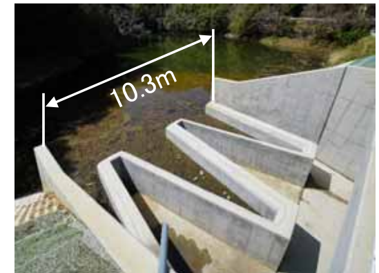
豪雨対策（洪水吐きの改修）の先行整備（例） ※地震対策は豪雨対策完了後に実施
