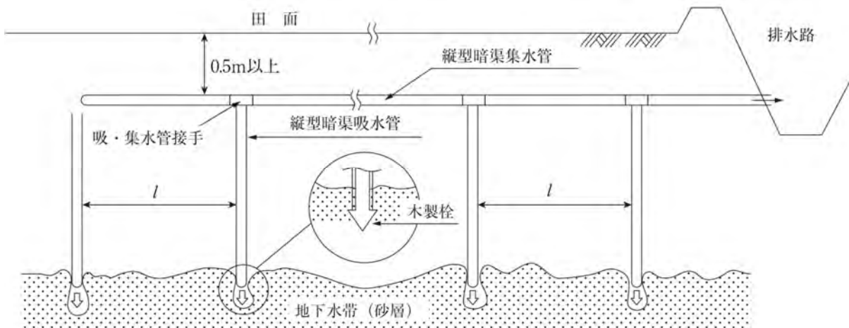
図-4.8.26 縦型暗渠の施工例
