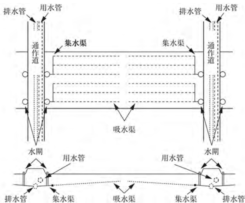
20 21 図-4.8.13 主な大区画水田の暗渠排水組織（両側へ排水する場合） 22
