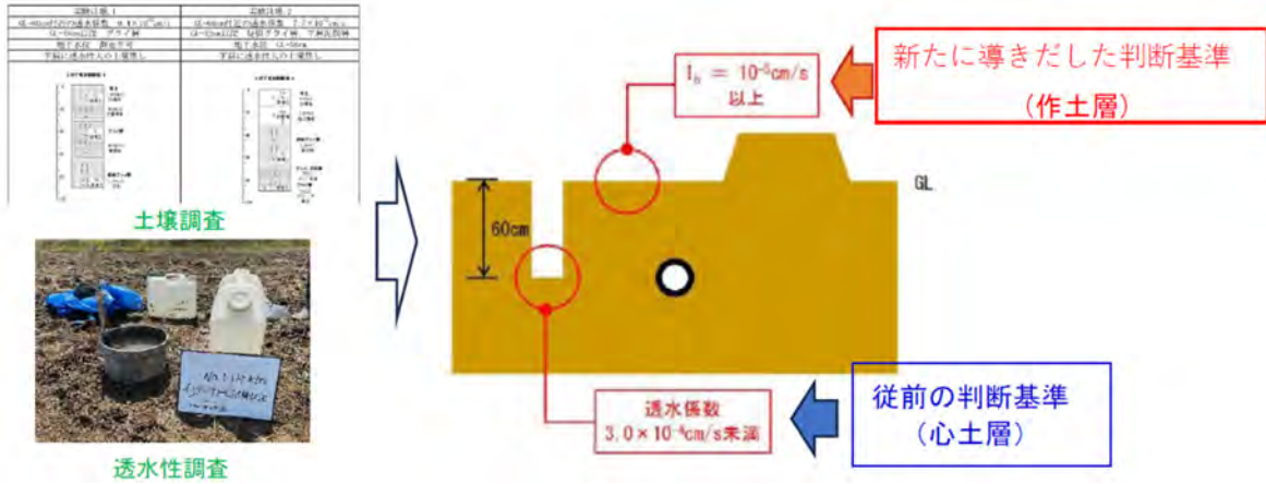
図-4.8.23 地下かんがいシステム導入の目安
