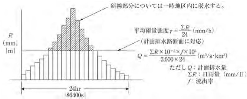
図-4.7.1 日雨量日排除の考え方
