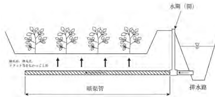
4 5 6 図-4.8.20 排水利用型
