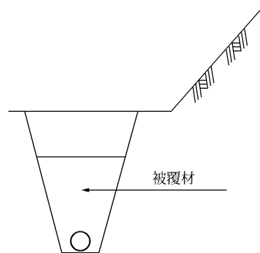
13 図-4.8.9 捕水渠の断面
