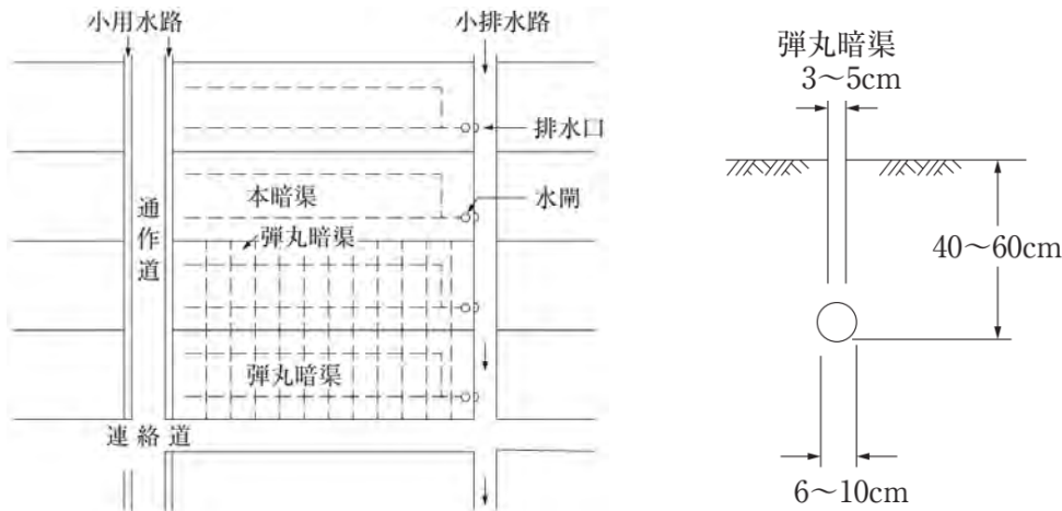
図-4.8.11 本暗渠と補助暗渠の組合せ設置例
