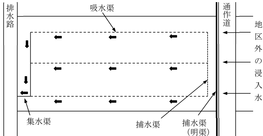
16 図-4.8.10 捕水渠、吸水渠、集水渠の配置例
