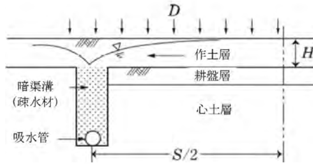
図-4.8.17 吸水渠構造の例
