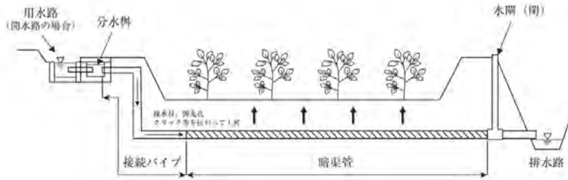
図-4.8.18 用水利用型
