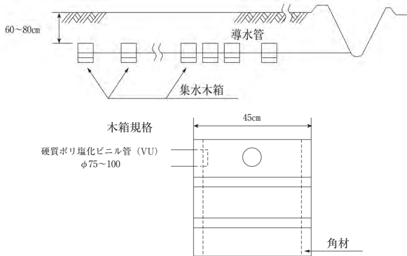
図-4.8.27 箱型暗渠の施工例
