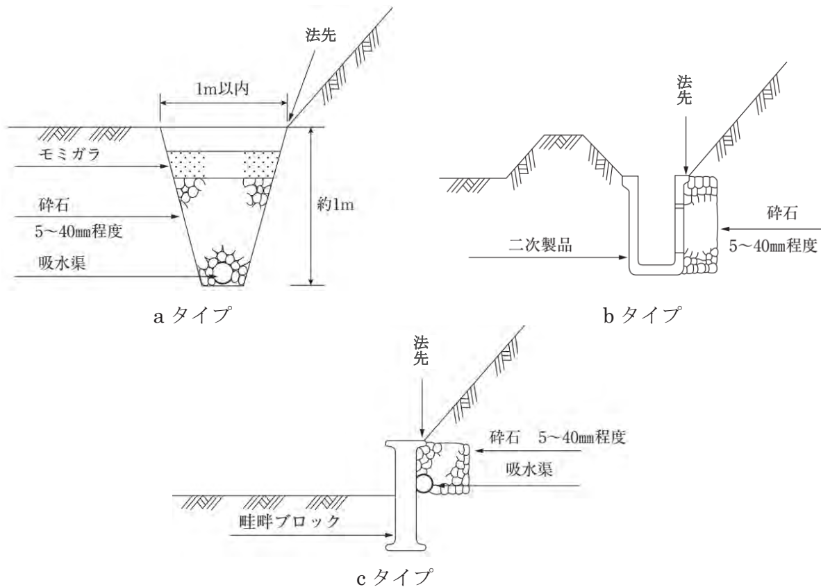
図-4.8.28 法先捕水渠の施工例
