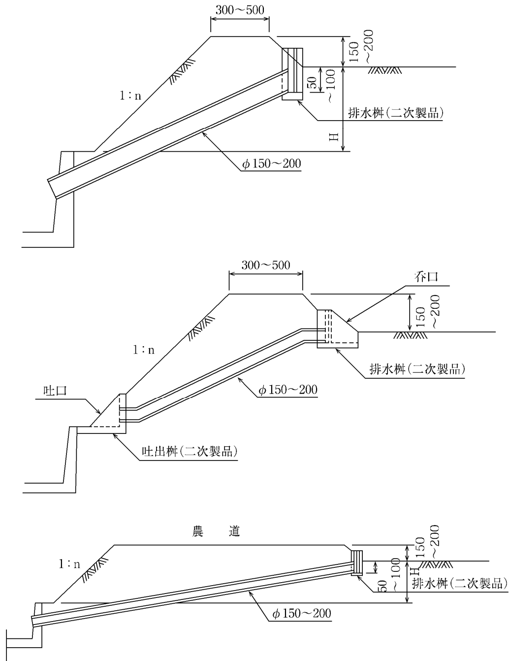
圖-4.7.10 落水口標準圖
