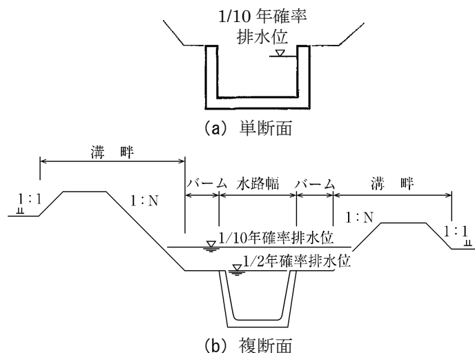
12 図-4.7.9 排水路標準断面図
