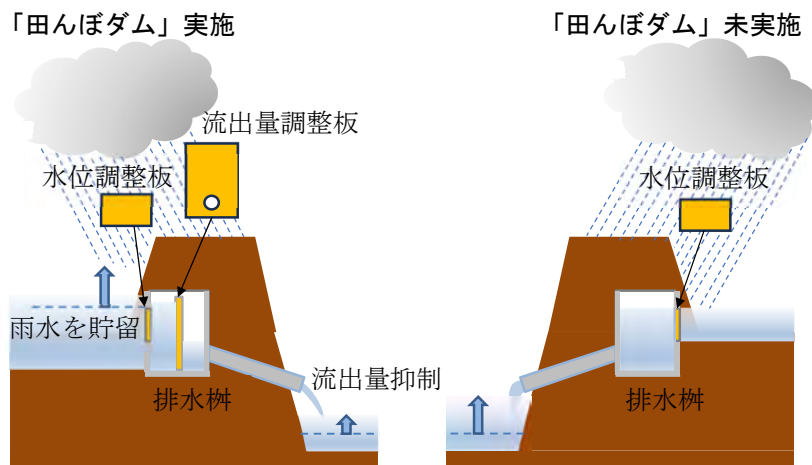
9 10 図-4.7.11 「田んぼダム」を実施している水田の排水イメージ 6)
