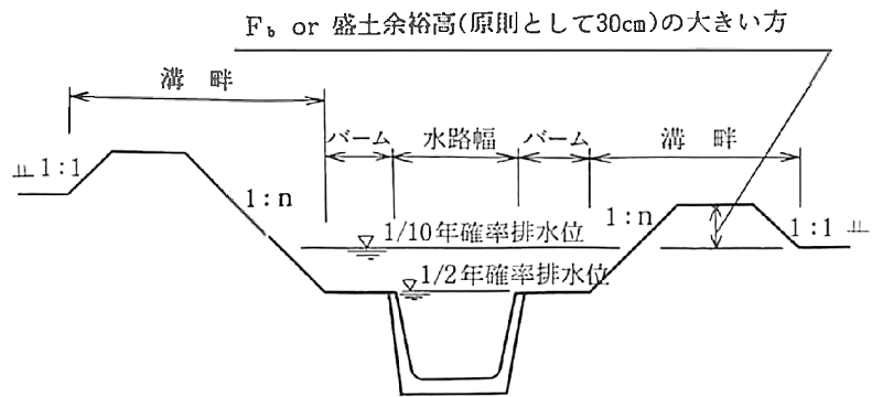
16 17 図-4.7.7 排水路（複断面）の余裕高
