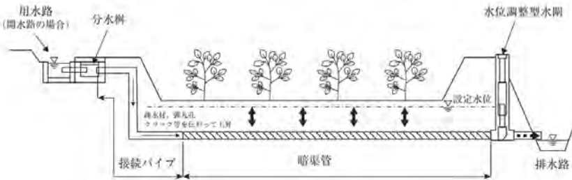
図-4.8.19 用水利用型 (地下水位制御型)
