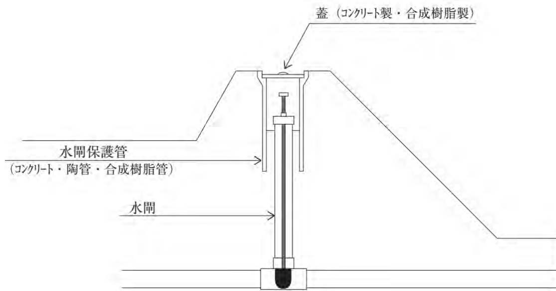
17 図-4.8.2 水閘保護管 18 19
