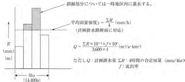
図-4.7.2 4時間雨量4時間排除の考え方
