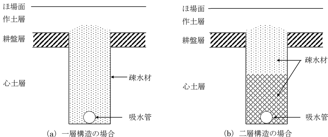
13 図-4.8.16 吸水渠構造の例
