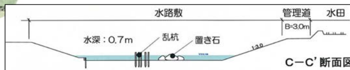
生態系保全型水路の概要
