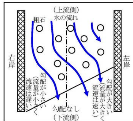
粗石付き片斜曲面式魚道による水の流れ (概略図)
