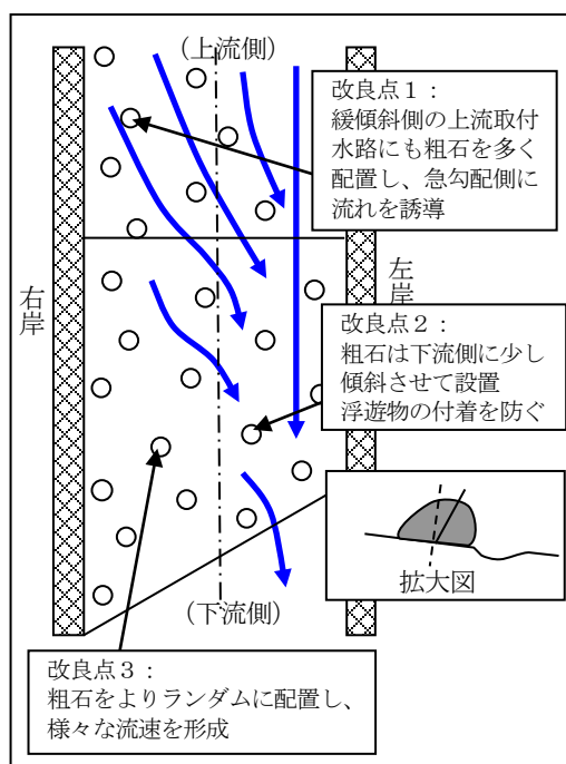
反省点を踏まえた改良点（概略図）
