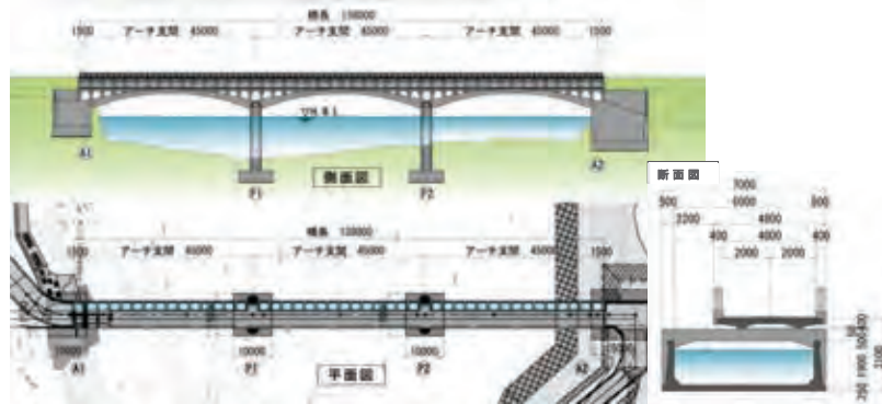
〔主要構造図（三面）〕
