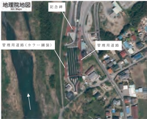
〔沈砂池の改修後の開放区間〕
