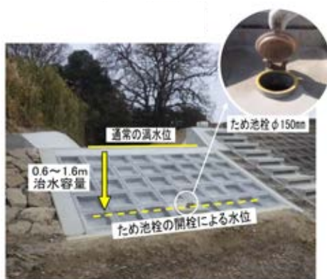
図-16.108 ため池栓の設置
