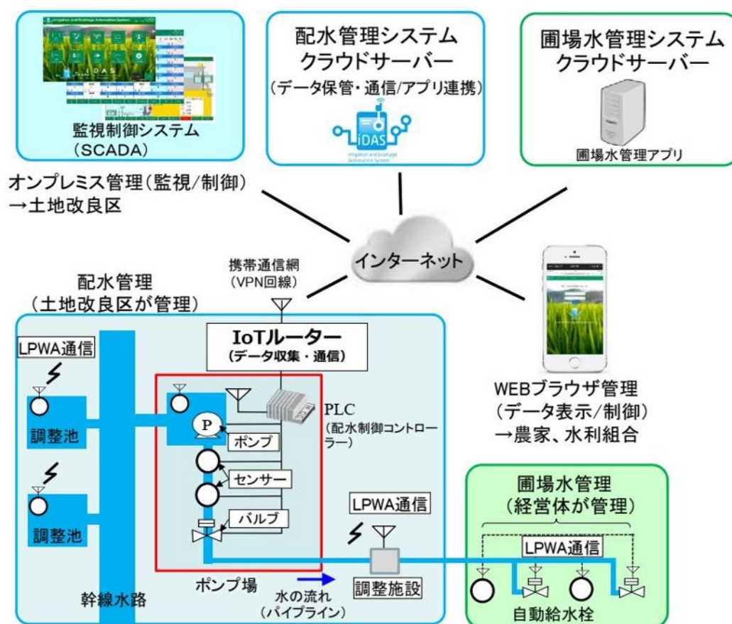
図-4.10.4 配水管理システムの構成 2)
