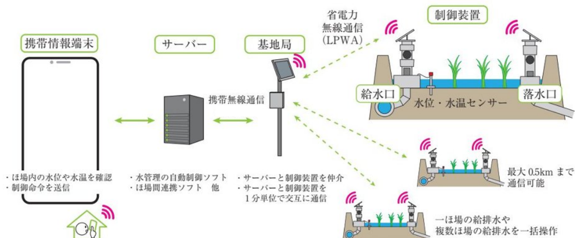
図-4.10.2 ほ場水管理システムの概要 2)
