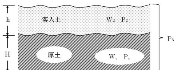
図-4.9.1 客土模式図
