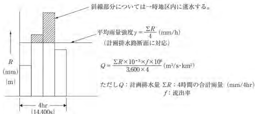
図-3.7.2 4 時間雨量 4 時間排除の考え方
