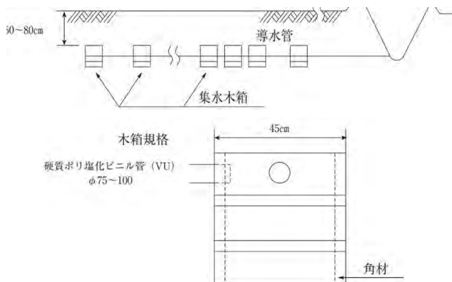
16 図-3.8.22 箱型暗渠の施工例
