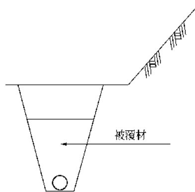
図-3.8.9 捕水渠の断面
