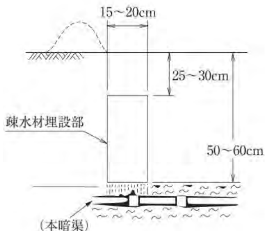
図-3.8.12 疎水材埋設暗渠大区画水田における暗渠排水組織
