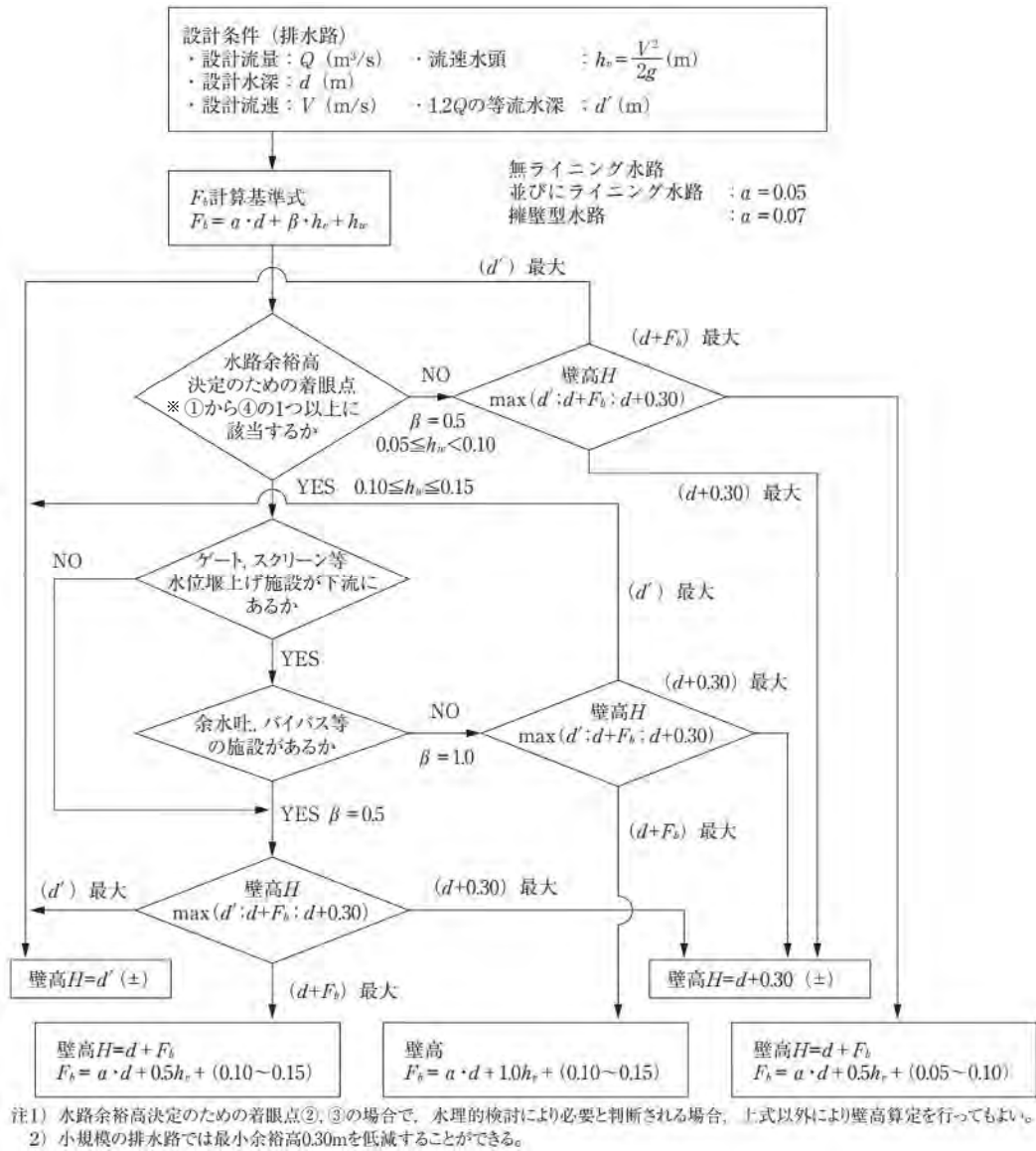
図-3.7.8 排水路（開水路）の余裕高算定と水路壁高決定のフローチャート
