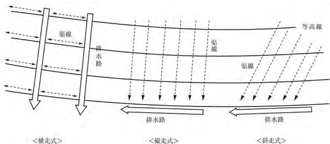
図-3.8.8 配置方式の分類
