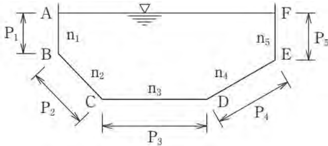
図-3.7.5 合成粗度係数の算定図
