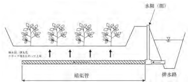
図-3.8.17 排水利用型
