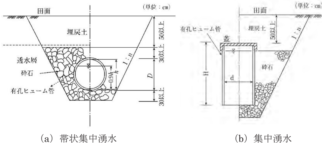
図-3.8.20 集水井型暗渠の施工例
