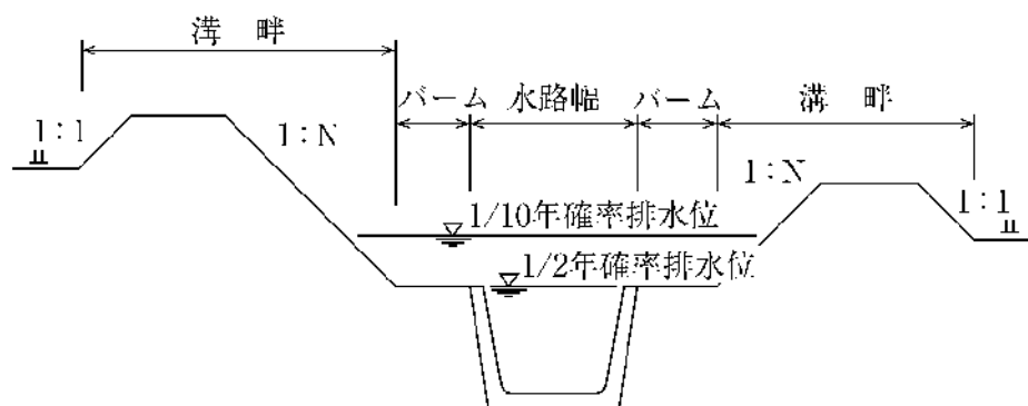
(b) 複断面
