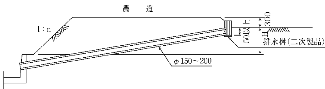
圖-3.7.10 落水口標準圖
