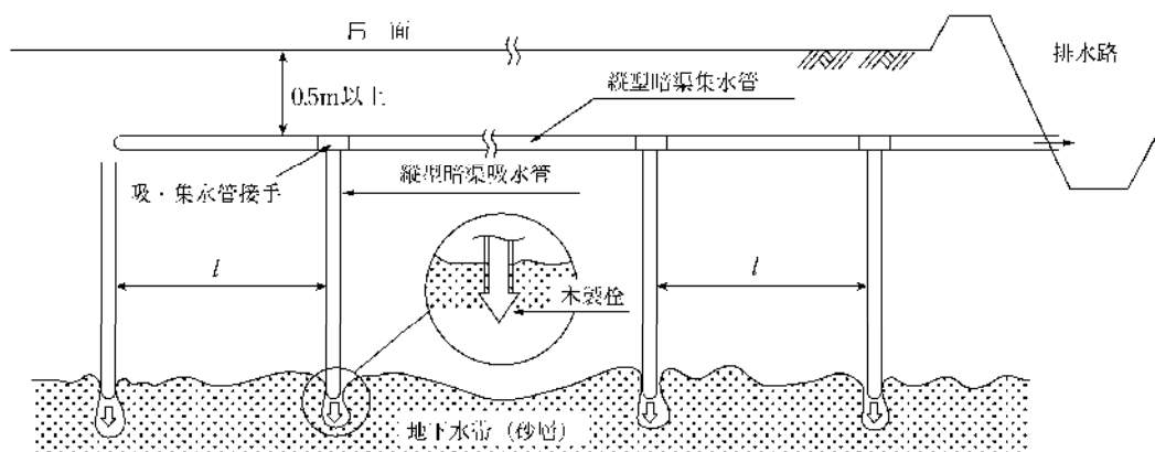
9 図-3.8.21 縦型暗渠の施工例
