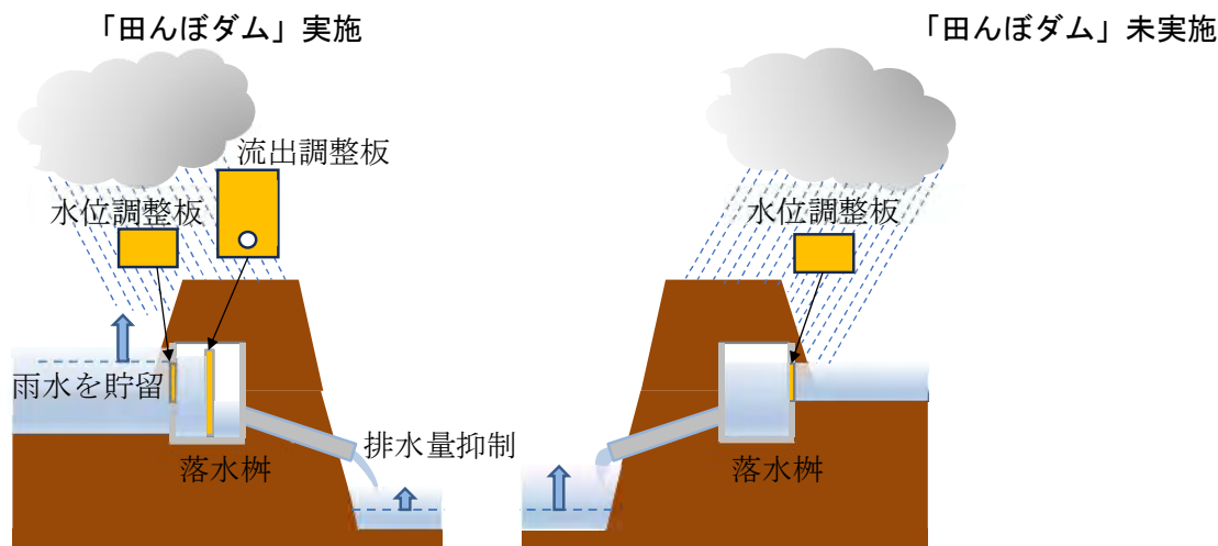
図-3.7.11 「田んぼダム」を実施している水田の排水イメージ
