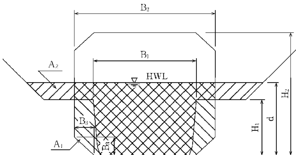
図-3.7.4 ボックスカルバートの通水断面
