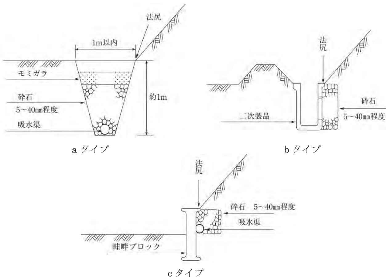
図-3.8.23 法先捕水渠の施工例
