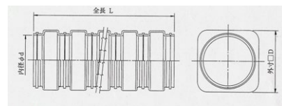
波付可とう電線管
