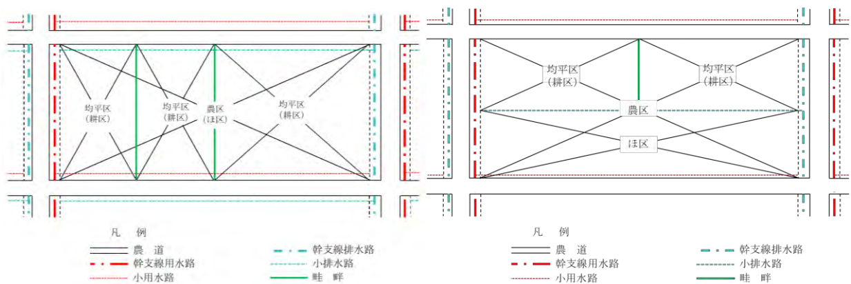
10 (a)農区の端に小排水路を配置する方法 (b)農区の中央に小排水路を配置する方法
