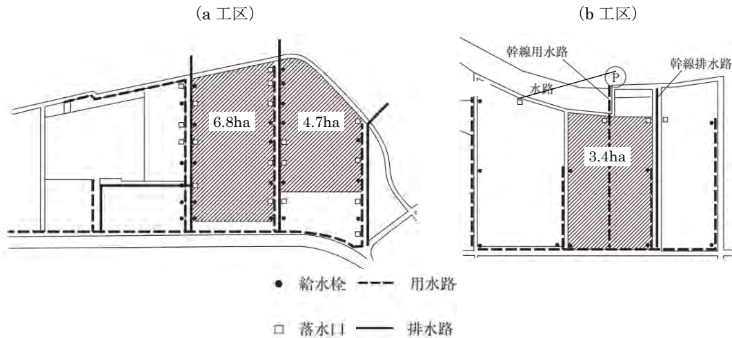
5 6 図-4.2.25 更なる大区画の整備事例 (B 地区)
