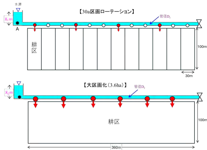
4 図-4.2.20 区画拡大後も 24 時間以内に給水する場合の給水状況の変化
