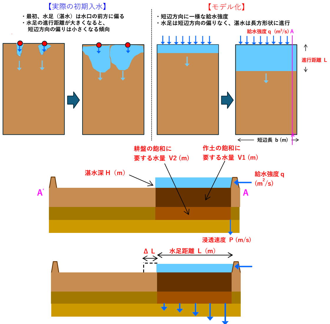
30 図-4.2.18 水足進行モデル
