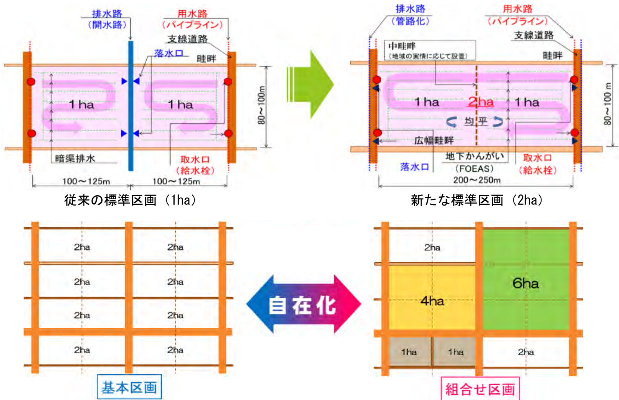
6 図-4.2.27 大区画及び更なる大区画の整備事例 (D 地区)
