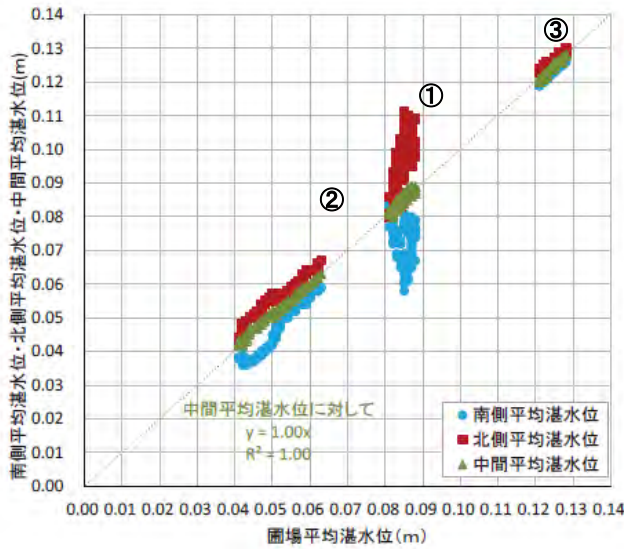
18 図-4.2.8 ほ場平均湛水位と地点ごとの平均湛水位
