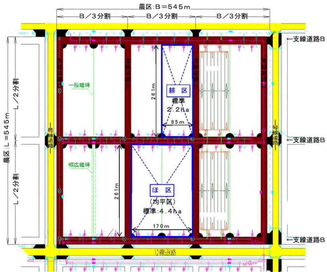
図-4.2.24 大区画の整備事例 (A 地区)
