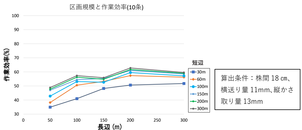
図-4.2.12 田植え作業における機械別の作業効率
