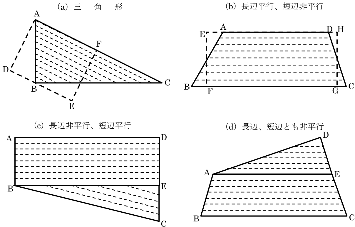
16 図-4.2.30 非方形区画
