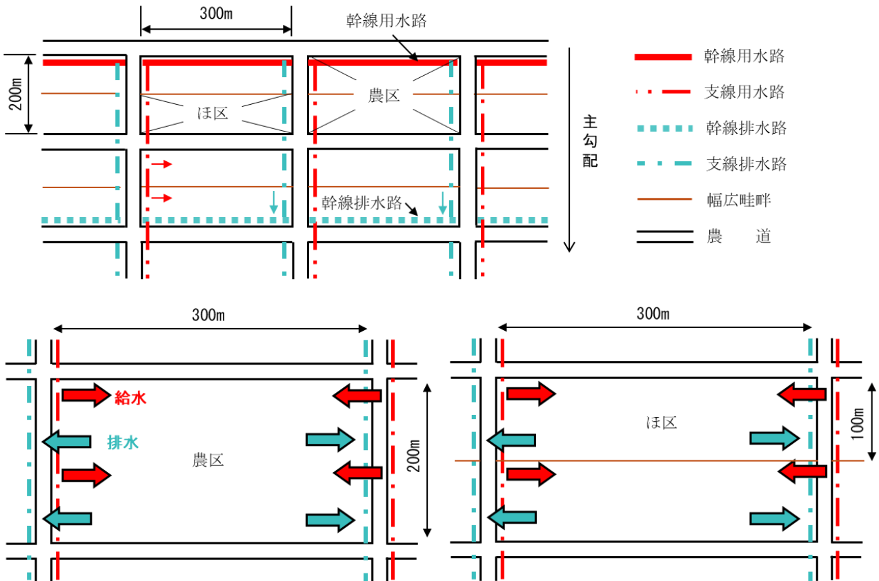
9 図-4.2.2 大区画化に向けた用排水路、農道の配置例
