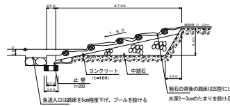
縦断面図 (B-B) 側部
