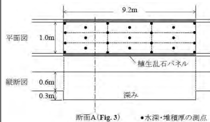
魚溜工の諸元
