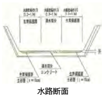
水路断面
