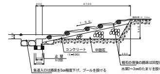
縦断面図 (B-B) 側部
