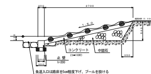
縦断面図 (A-A) 流芯部
