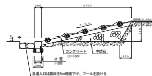
縦断面図 (A-A) 流芯部
