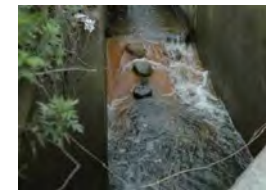
改良された魚道（片斜面粗石付魚道）
